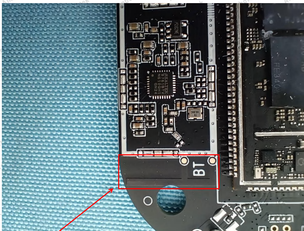
BT&BLE ANT
