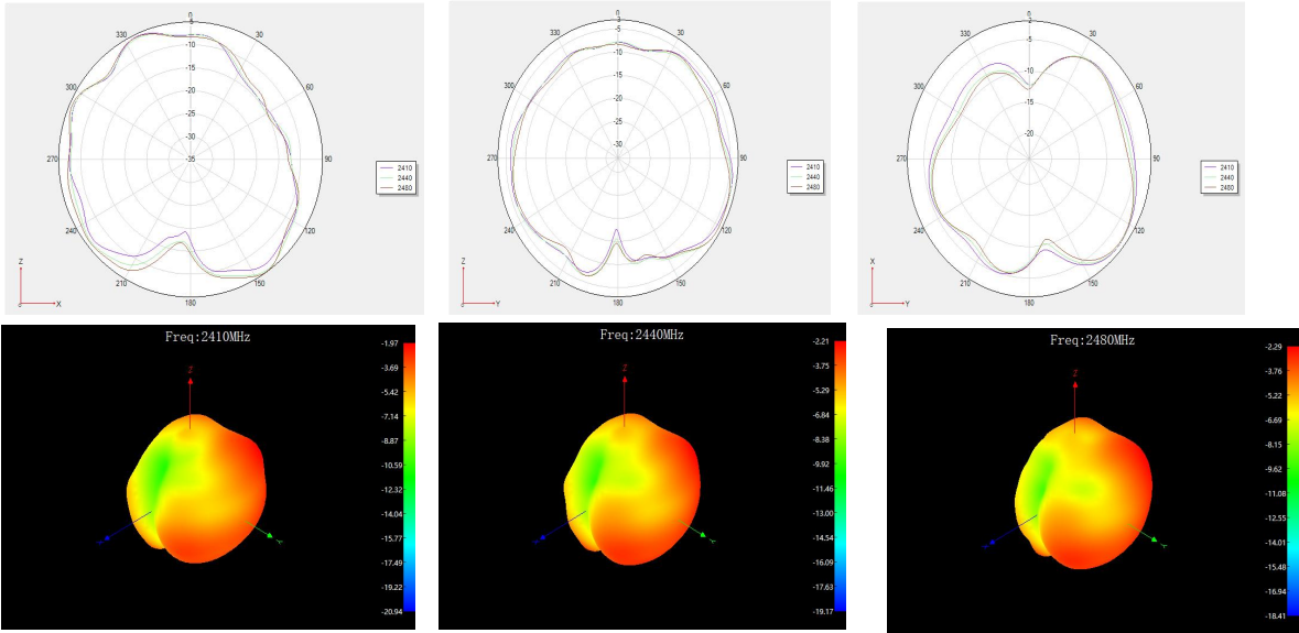
无源方向图
