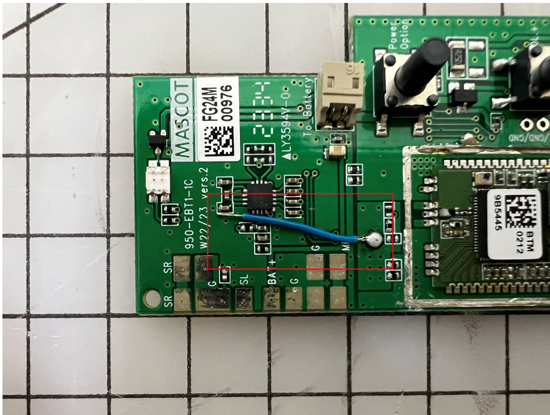
EUT-6. Antenna
