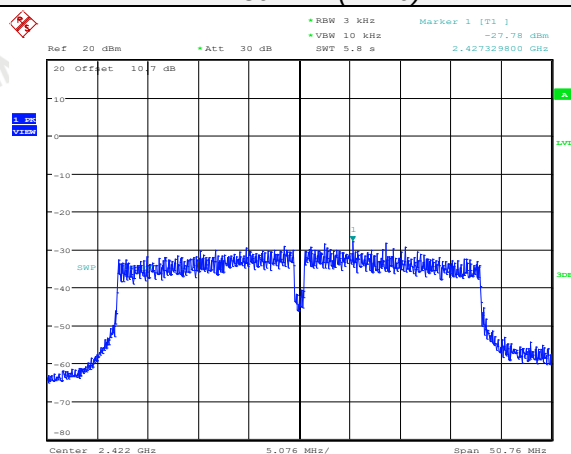
802.11n(HT40)
