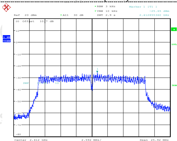
802.11n(HT20)
