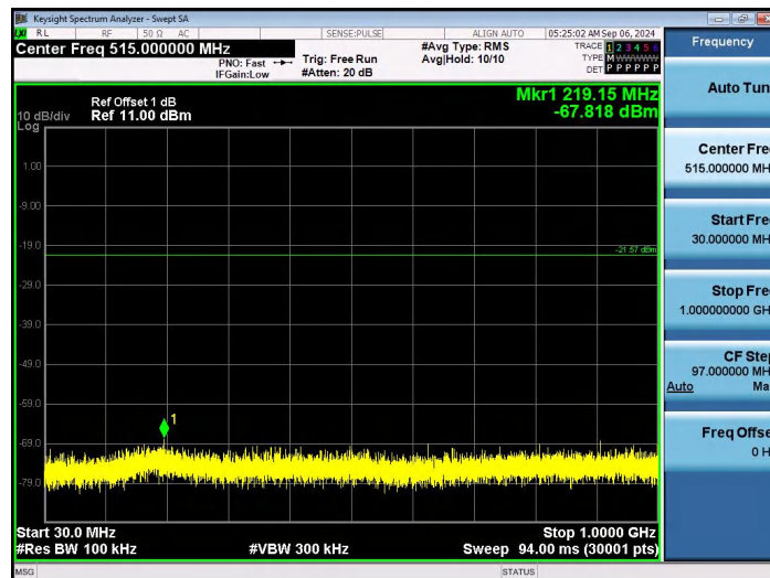
BLE_2M-Ant1-2480-30~1000-PASS
