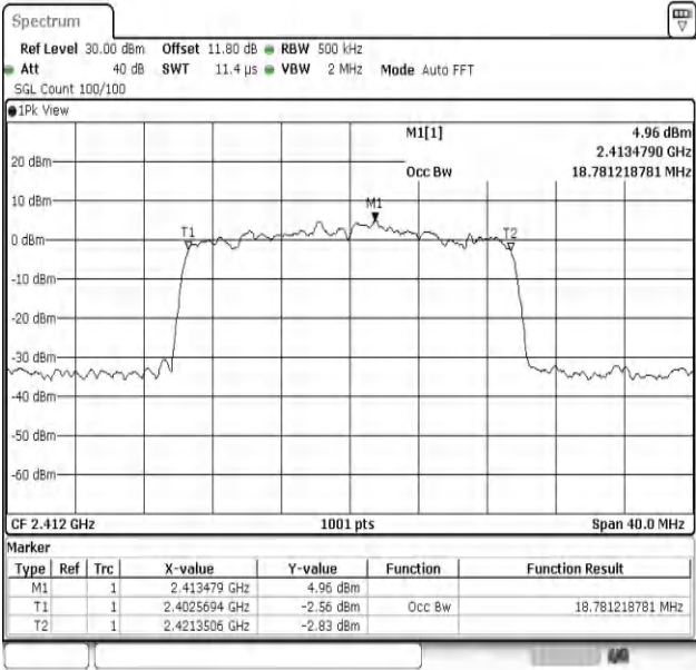
11AX20MIMO-Ant2-2412
