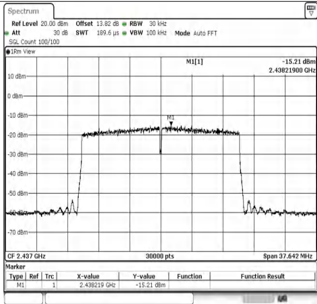
11AX20MIMO-Ant1-2437-PASS
