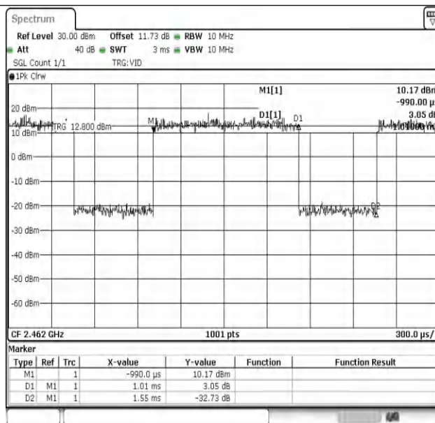
NTNV-11AX20MIMO-Ant1-2462
