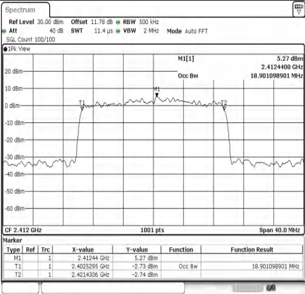
11AX20MIMO-Ant1-2412
