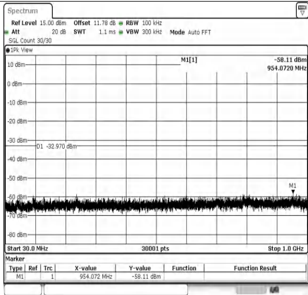
11G-Ant1-2412-30~1000-PASS
