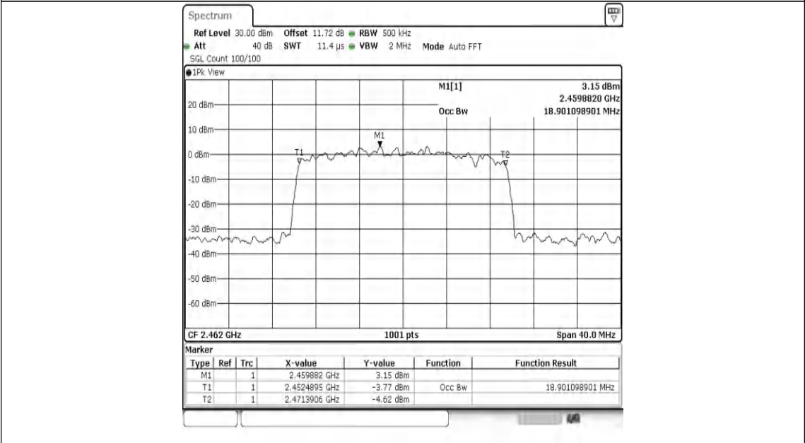
11AX20MIMO-Ant2-2462
