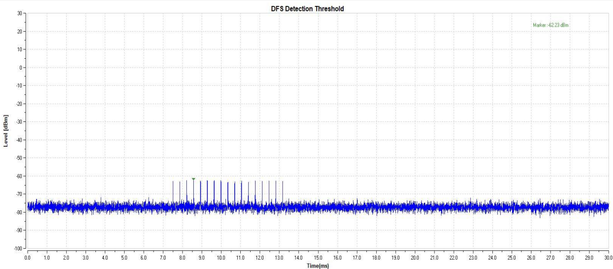
11AC40-5270-Type3-PASS
