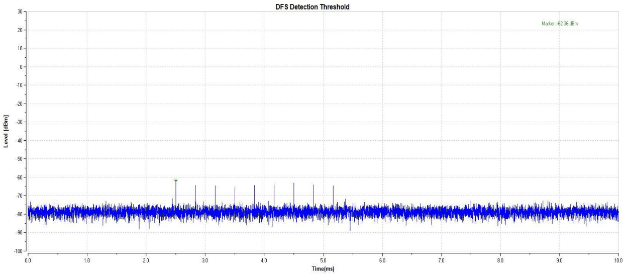
11AC40-5270-Type6-PASS
