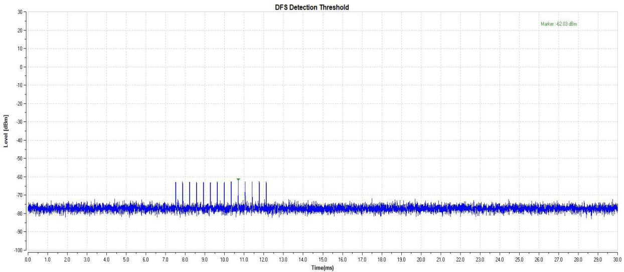
11AC40-5270-Type4-PASS
