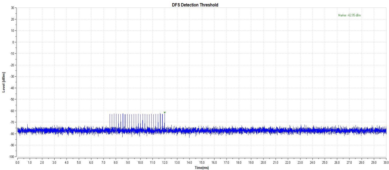
11AC40-5270-Type2-PASS
