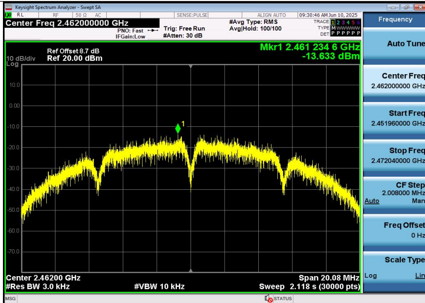
11B-Ant2-2462-PASS
