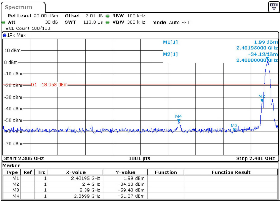
Band Edge BLE 2M 2402MHz Emission
