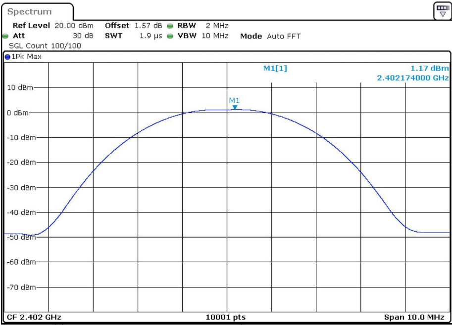
Power BLE 1M 2402MHz
