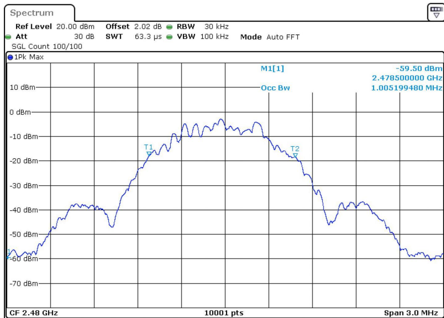
OBW BLE 1M 2480MHz
