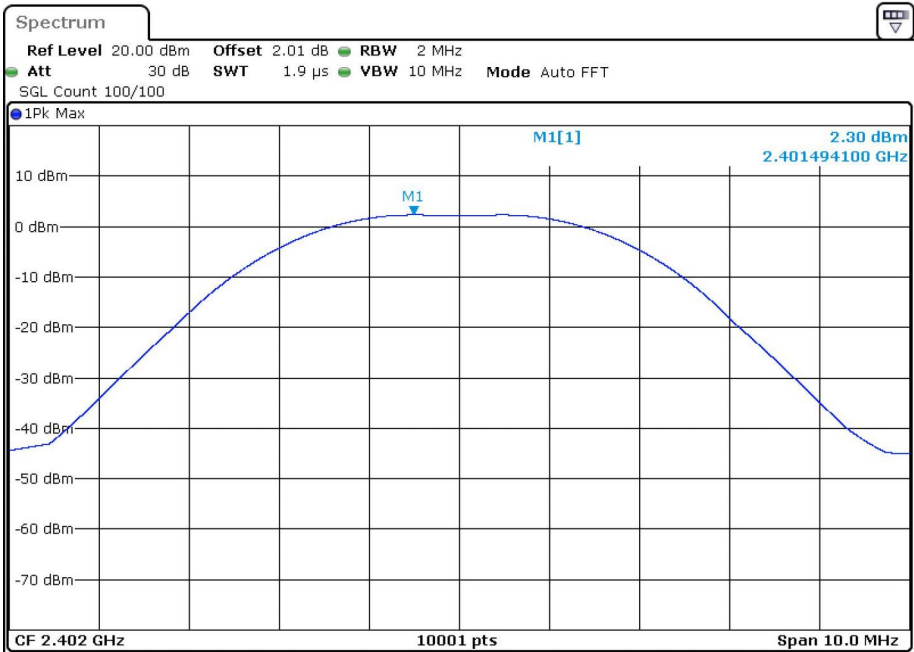
Power BLE 2M 2402MHz
