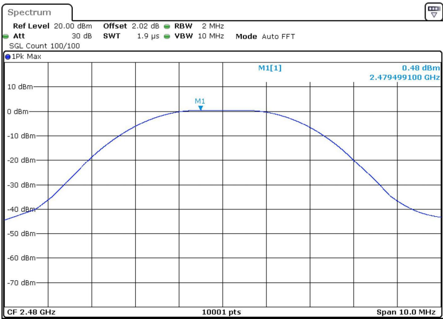
Power BLE 2M 2480MHz
