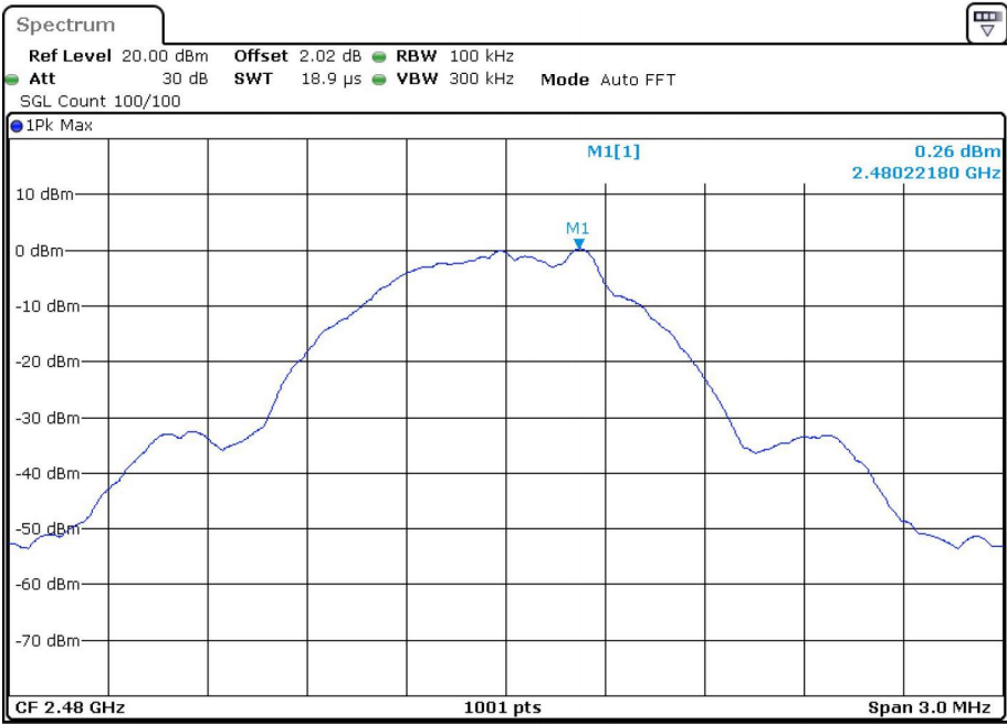
PSD BLE 1M 2480MHz
