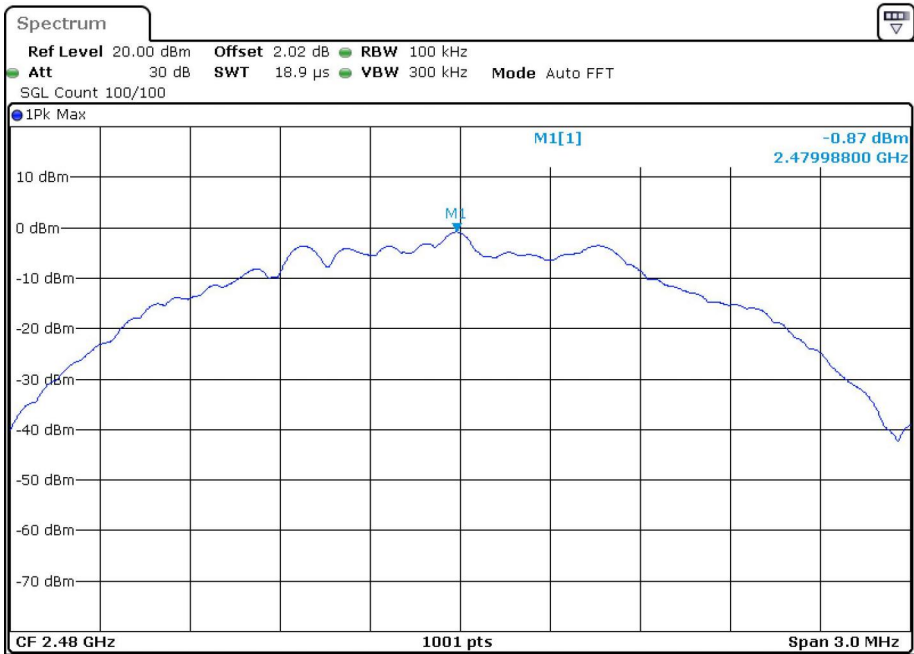
PSD BLE 2M 2480MHz
