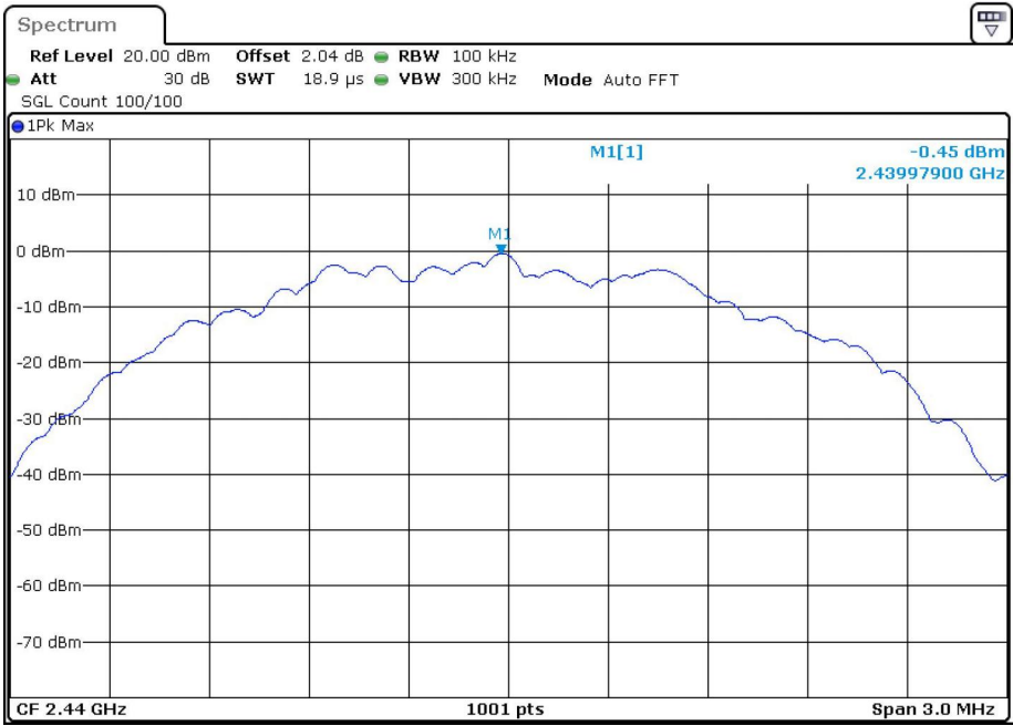
PSD BLE 2M 2440MHz
