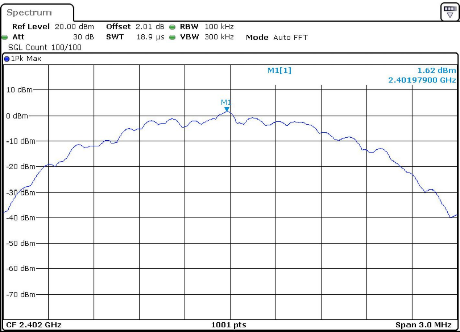
PSD BLE 2M 2402MHz
