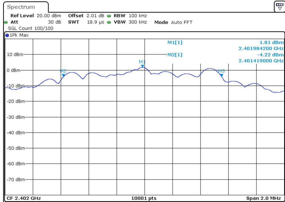
-6dB Bandwidth BLE 2M 2402MHz
