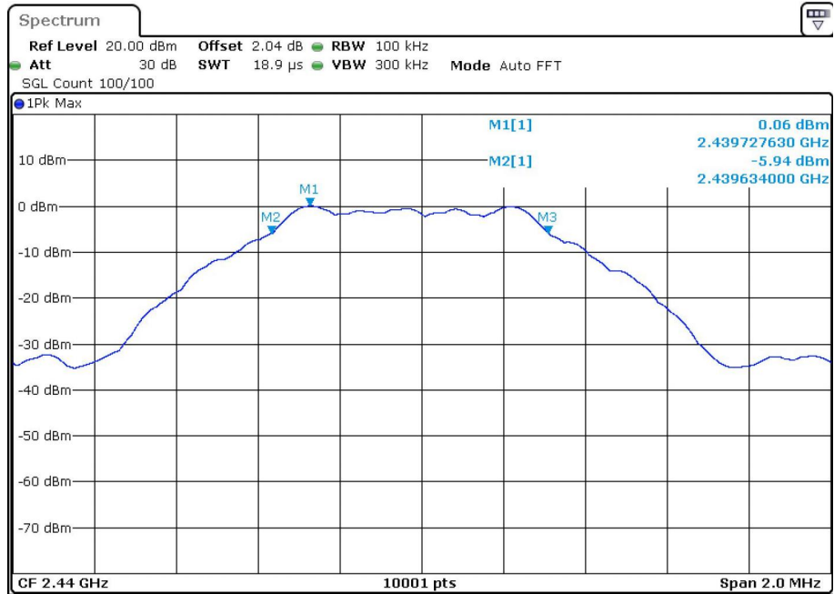
-6dB Bandwidth BLE 1M 2440MHz
