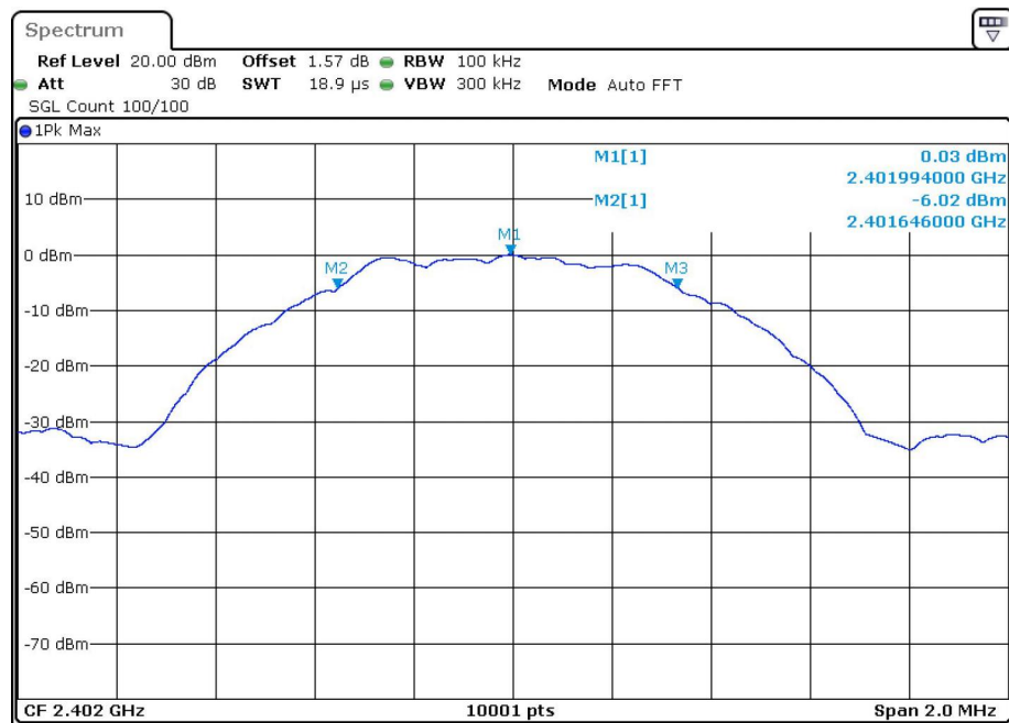
-6dB Bandwidth BLE 1M 2402MHz
