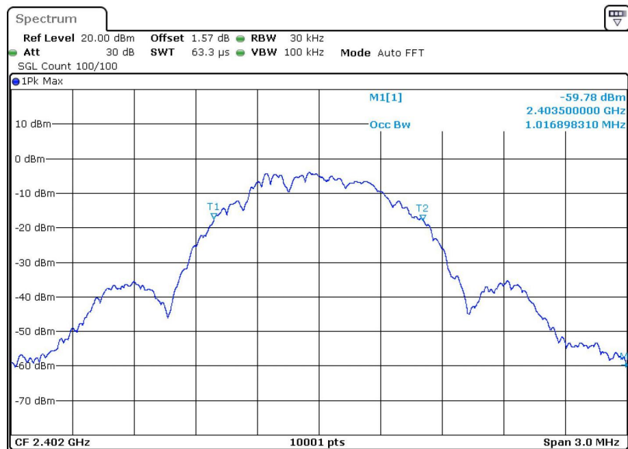
OBW BLE 1M 2402MHz
