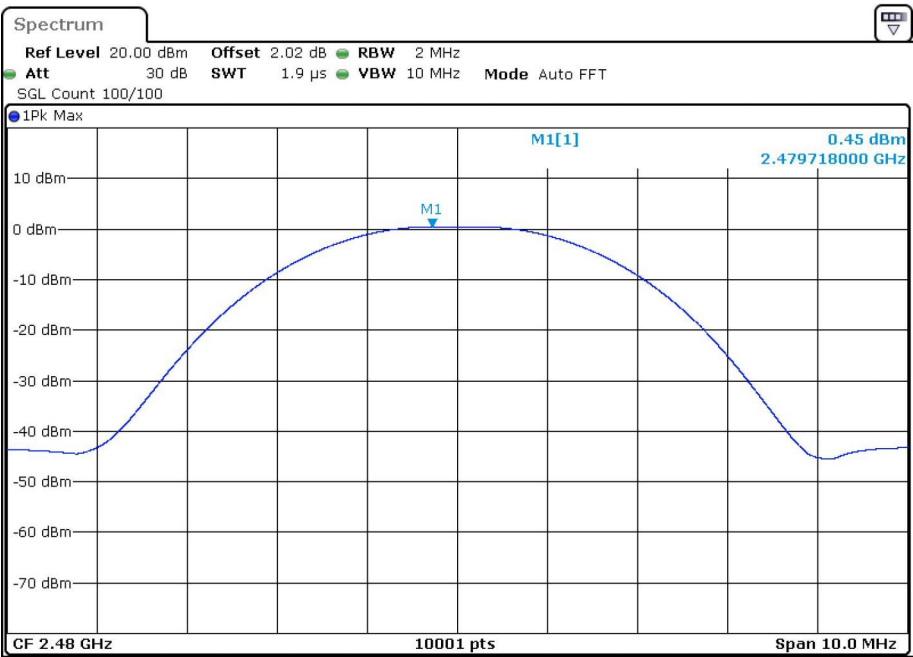
Power BLE 1M 2480MHz
