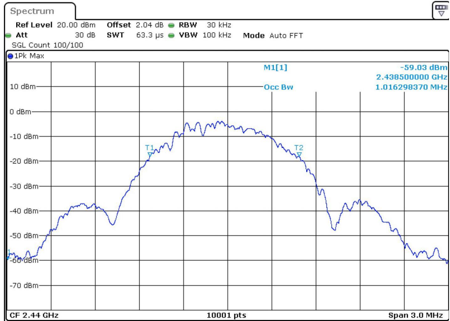
OBW BLE 1M 2440MHz
