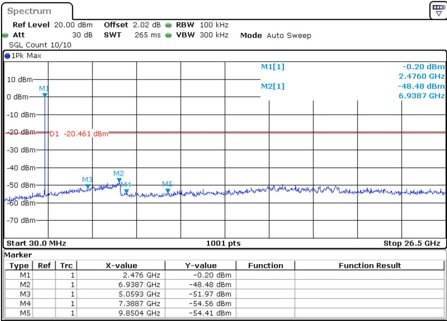
Tx. Spurious BLE 2M 2480MHz Emission
