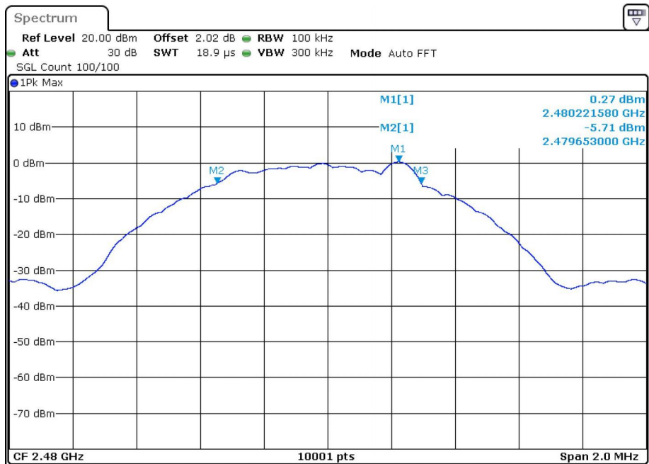
-6dB Bandwidth BLE 1M 2480MHz
