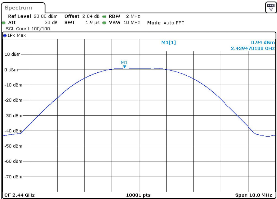
Power BLE 2M 2440MHz
