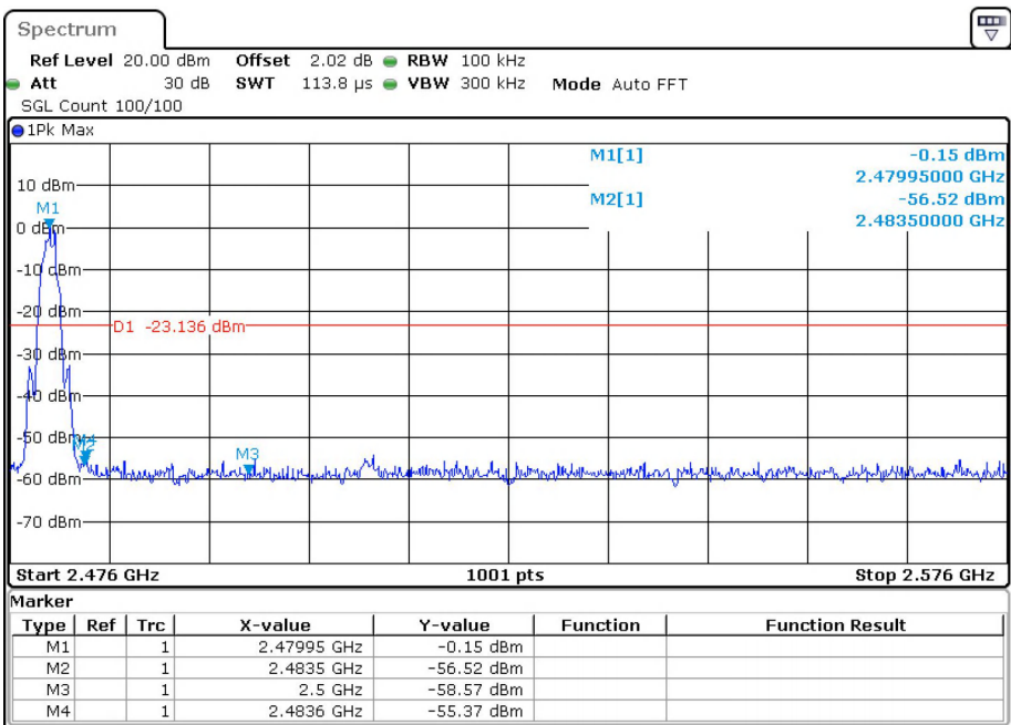
Band Edge BLE 2M 2480MHz Emission
