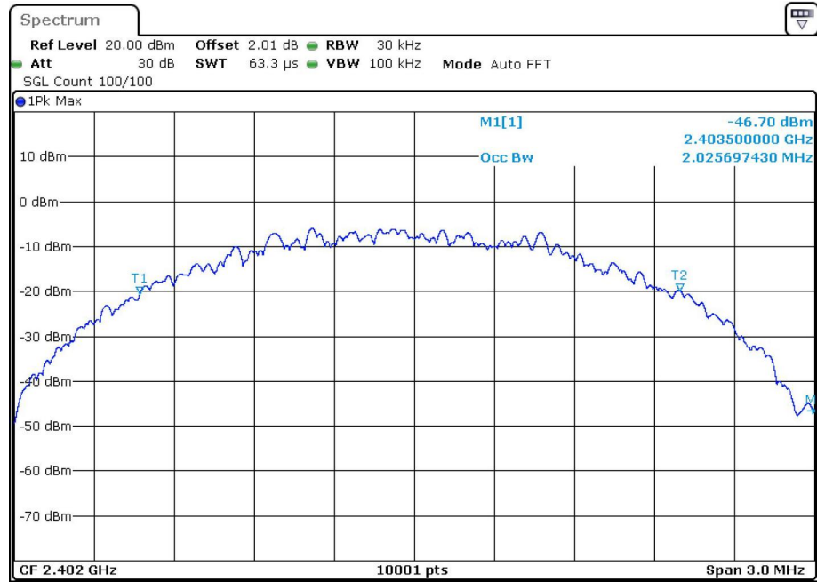
OBW BLE 2M 2402MHz
