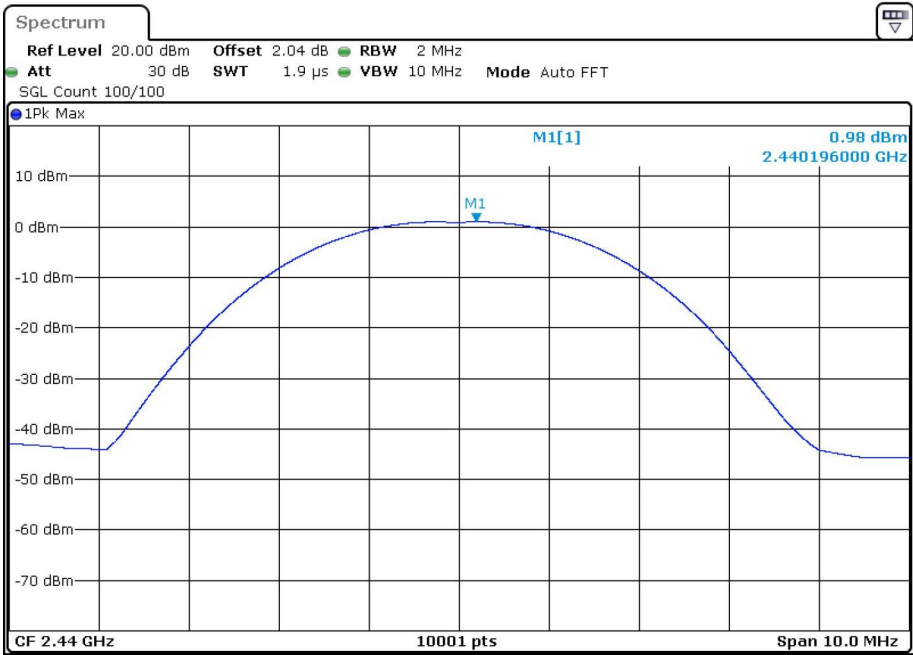
Power BLE 1M 2440MHz
