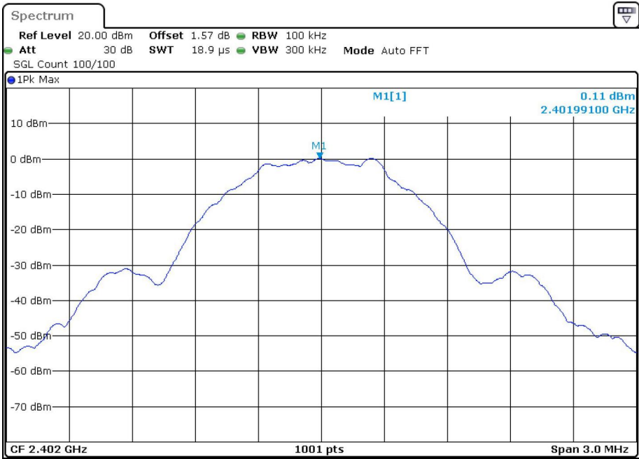
PSD BLE 1M 2402MHz
