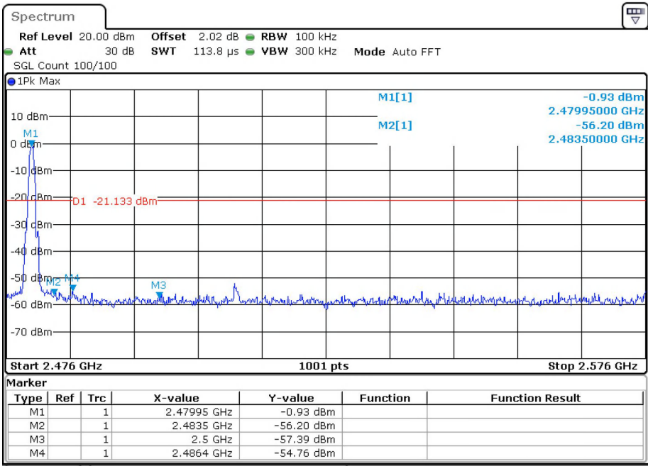
Band Edge BLE 1M 2480MHz Emission
