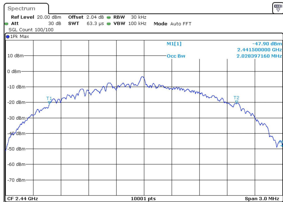
OBW BLE 2M 2440MHz
