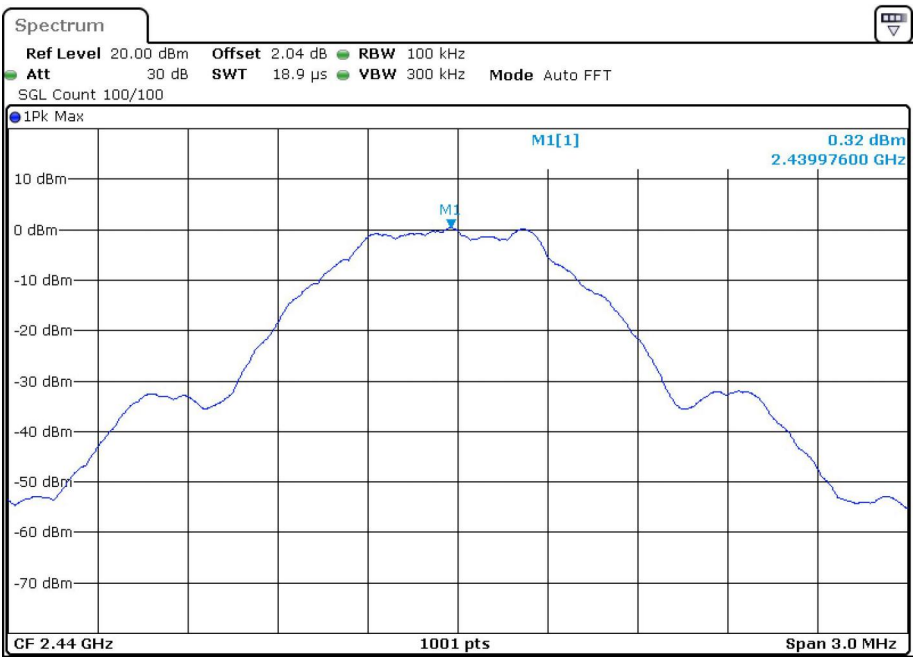
PSD BLE 1M 2440MHz
