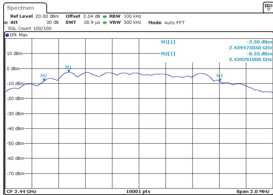
-6dB Bandwidth BLE 2M 2440MHz
