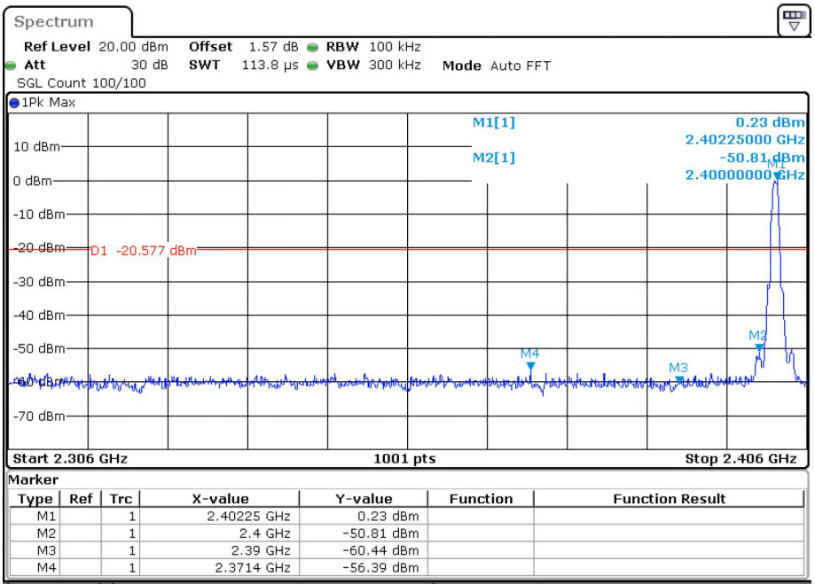
Band Edge BLE 1M 2402MHz Emission
