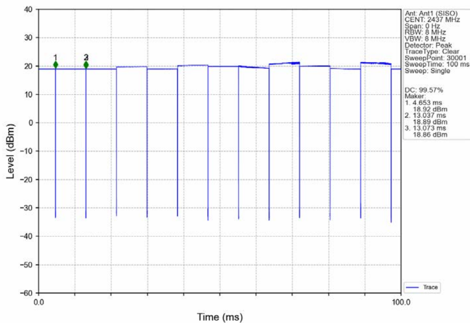
802.11b_MCH_2437MHz_Ant1 (SISO)_NTNV
