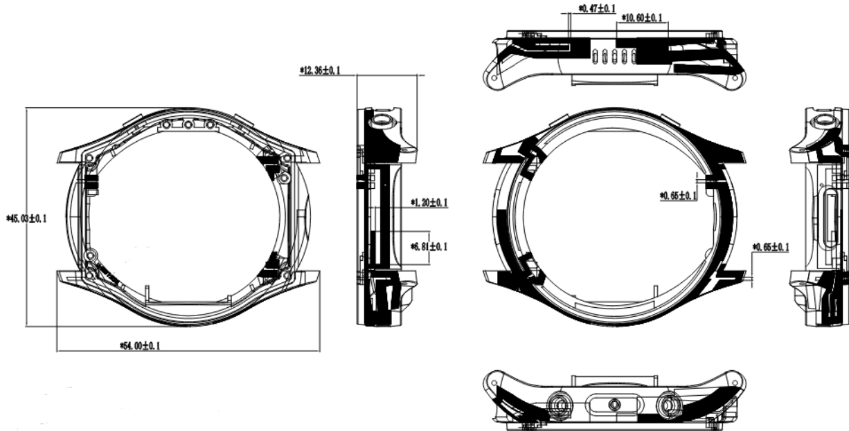
4G Antenna
