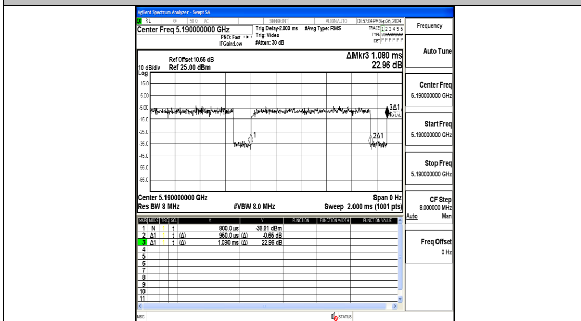
NTNV-11N40MIMO-Ant1-5190
