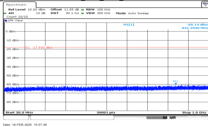
SRD 2.4G_Ant1_2480_30-1000
