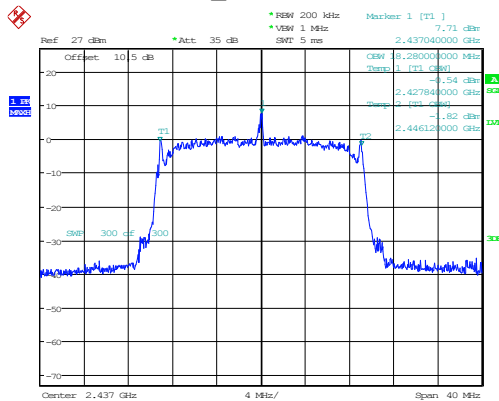
802.11n20_2437MHz 18.280MHz
