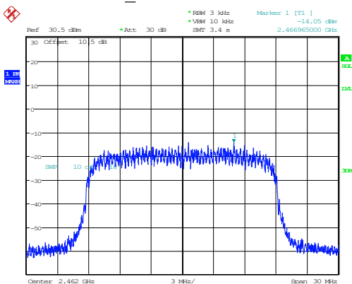
802.11n20_2462MHz -14.05dBm/3kHz
