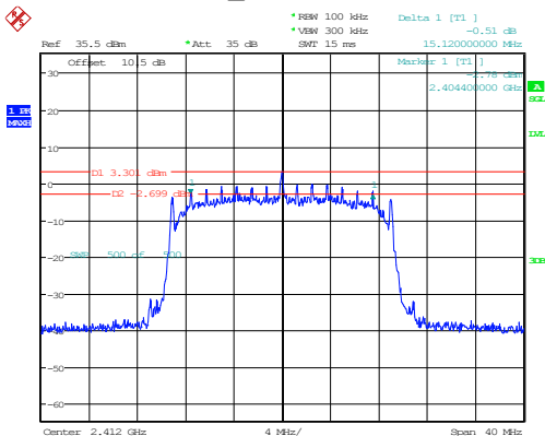
802.11n20_2412MHz 15.120MHz
