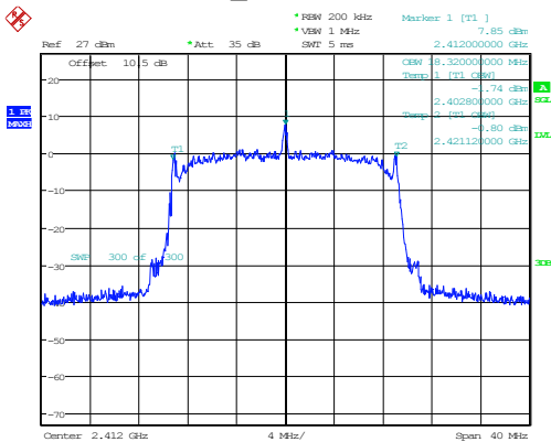
802.11n20_2412MHz 18.320MHz
