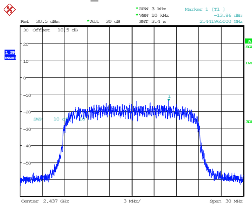
802.11n20_2437MHz -13.86dBm/3kHz
