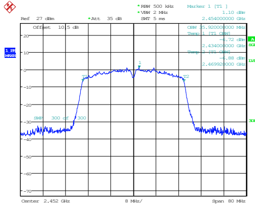
802.11n40_2452MHz 35.920MHz
