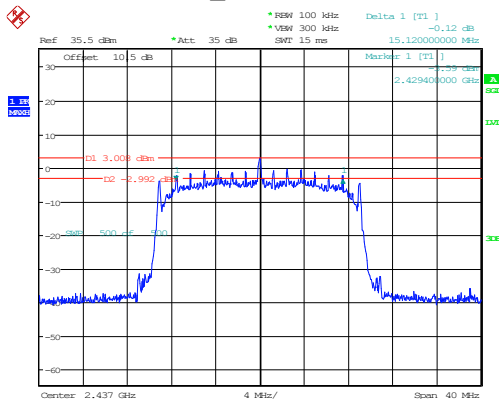
802.11n20_2437MHz 15.120MHz
