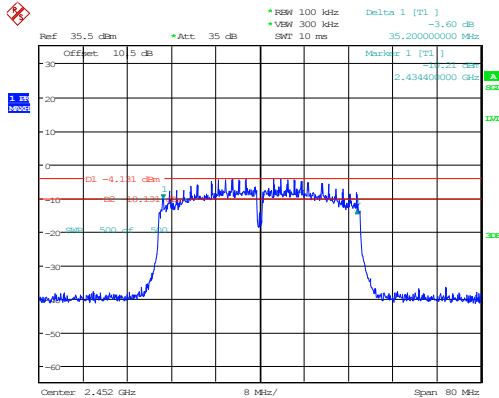
802.11n40_2452MHz 35.200MHz
