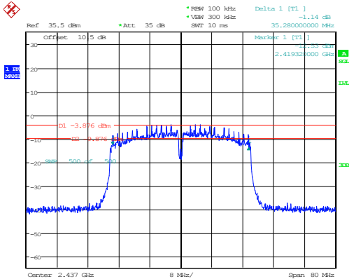
802.11n40_2437MHz 35.280MHz
