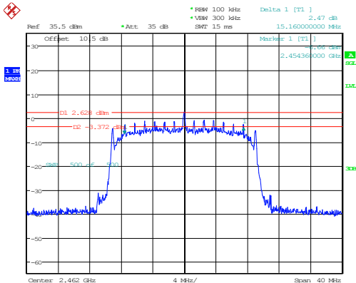
802.11n20_2462MHz 15.160MHz
