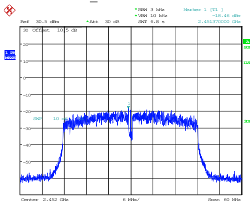
802.11n40_2452MHz -18.46dBm/3kHz
