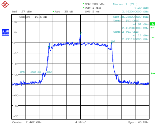
802.11n20_2462MHz 18.280MHz
