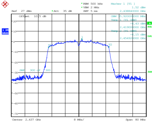
802.11n40_2437MHz 35.920MHz
