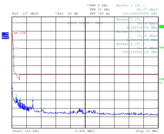
150kHz-30MHz
