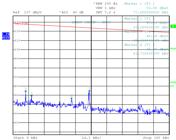
9kHz-150kHz
