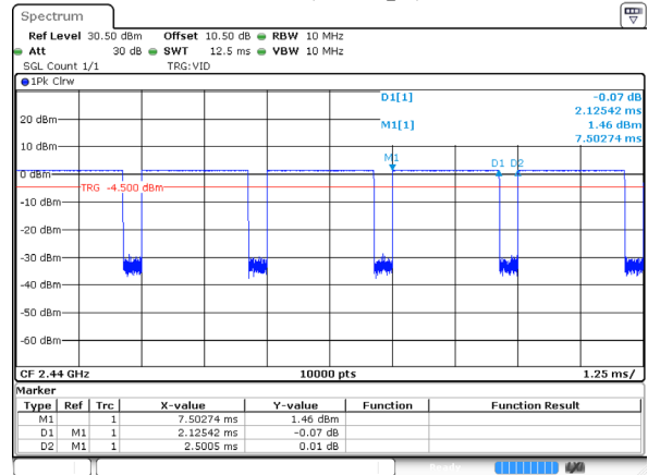
BLE (1 Mbps)
