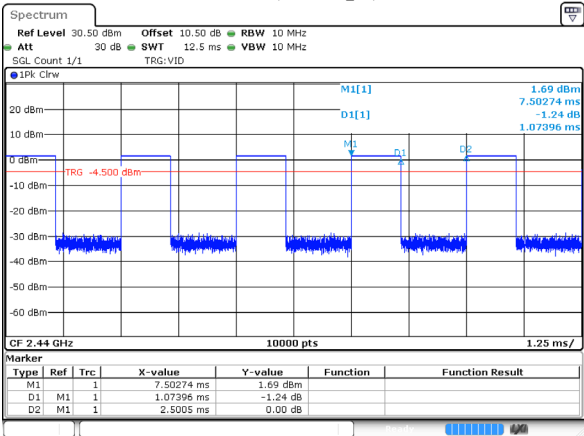
BLE (2 Mbps)
