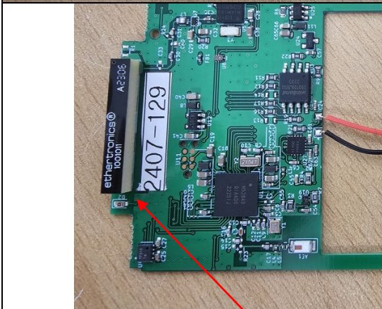
GPS Antenna
