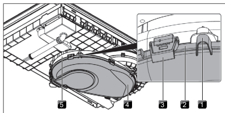
Fig. 9.3 Boîtier de circulation de l'air
