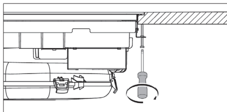
Fig. 11.18 Fixation sécurisée de la table de cuisson
