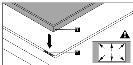
Fig. 11.16 Positionnement des plaques de compensation des hauteurs
