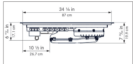
Fig. 5.5 Vue avant
