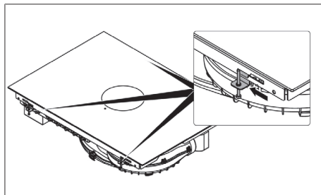
Fig. 11.14 Ajustement des brides de montage
