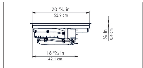
Fig. 5.6 Vue latérale
