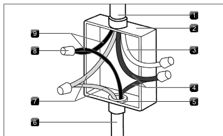
Fig. 11.20 Câble 4 fils
