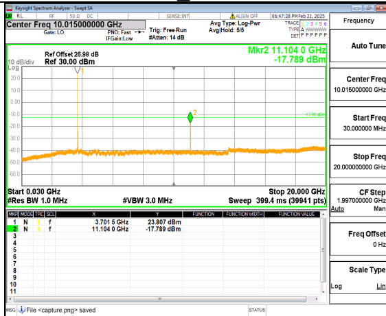
12A_n77(3700-3980MHz) (30MHz-20GHz) 20M DFT-s-OFDM QPSK Inner_1RB_Left Low
