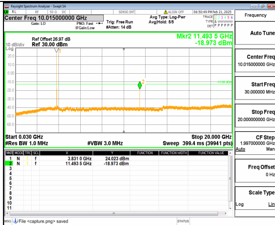
12A_n77(3700-3980MHz) (30MHz-20GHz) 20M DFT-s-OFDM QPSK Inner_1RB_Left Mid
