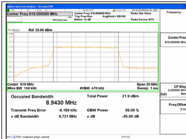
B26 Part90 / 10MHz / 64QAM/ Mid CH
