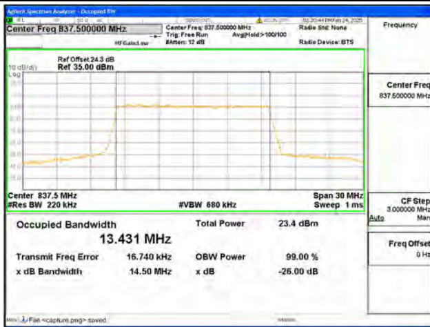
B19 / 15MHz / QPSK / Mid CH
