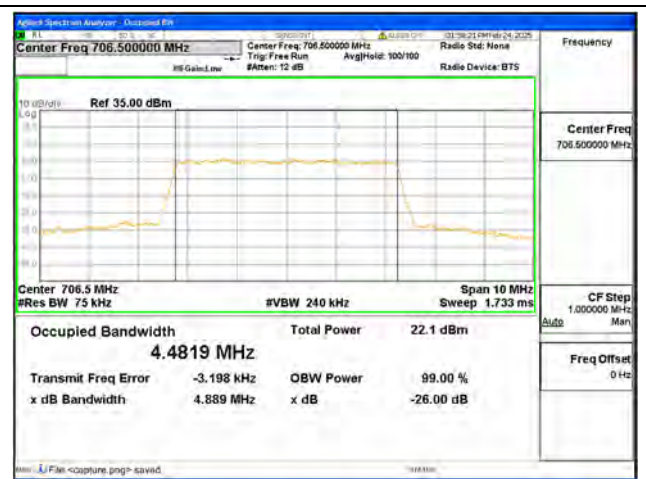
B17 / 5MHz / 16QAM/ Low CH
