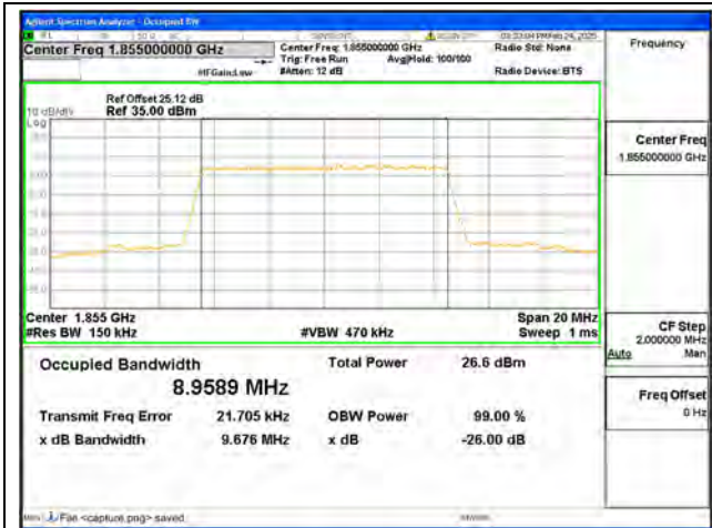
B25 / 10MHz / QPSK / Low CH
