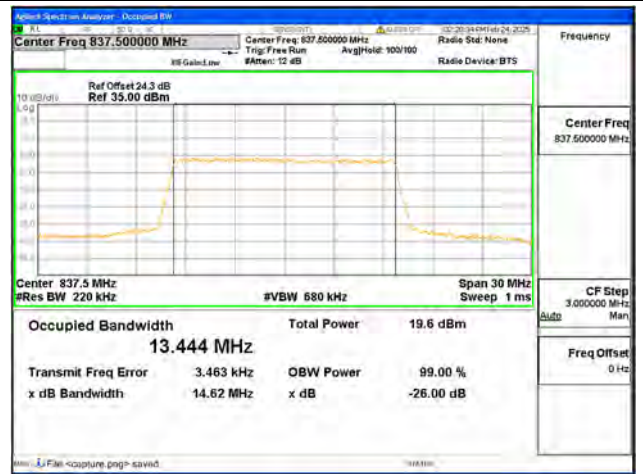
B19 / 15MHz / 256QAM / Low CH
