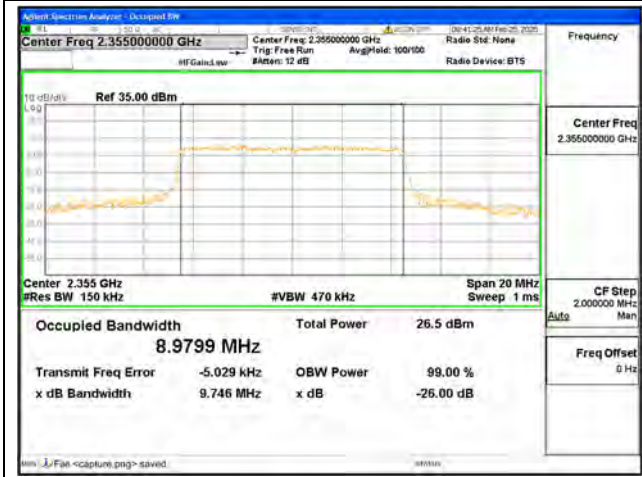
B40-2 / 10MHz / 64QAM / Mid CH
