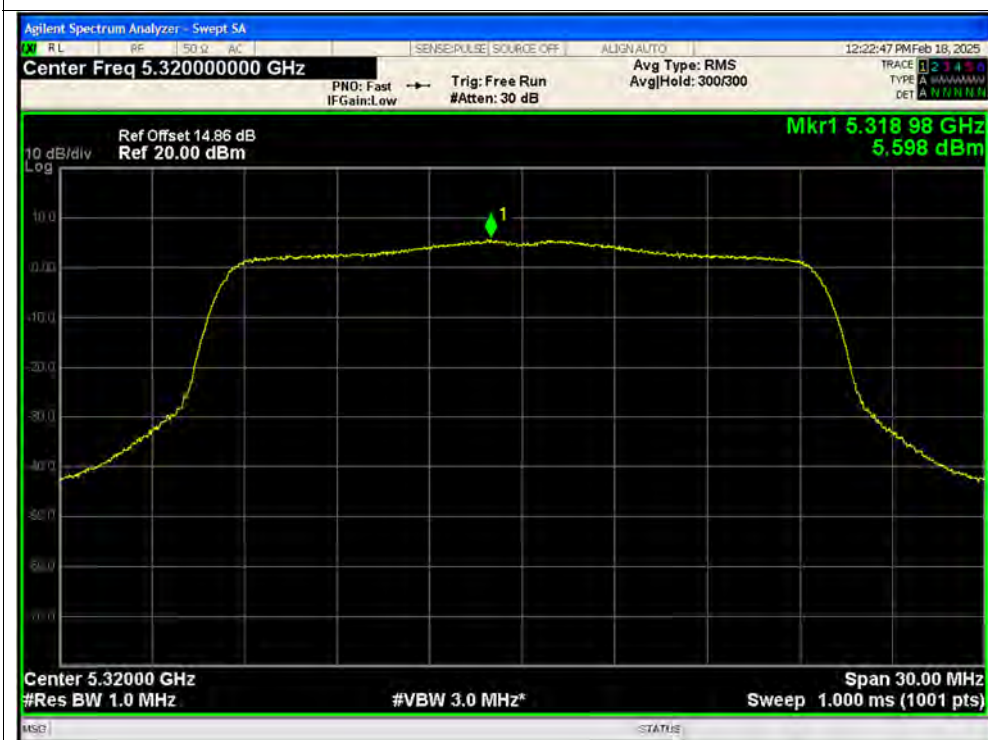
PSD NVNT ax20 5320MHz Ant1 SISO
