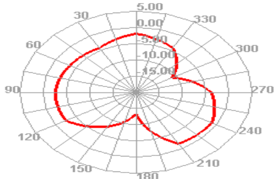
2400.000MHz E1
