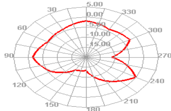
2400.000MHz E2
