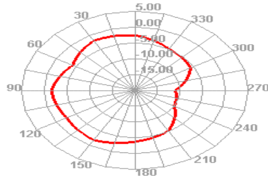
2400.000MHz H
