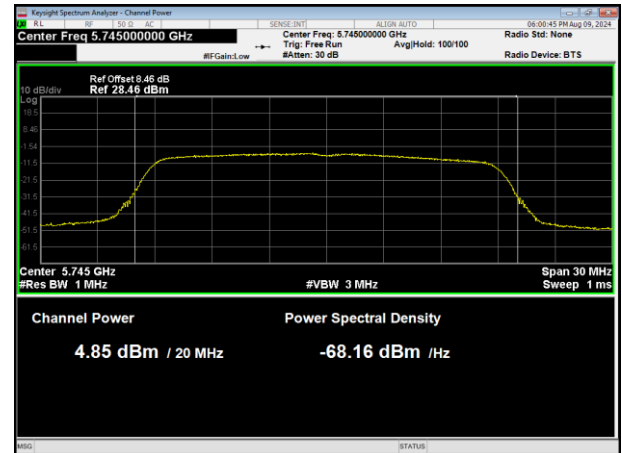
5745MHz
