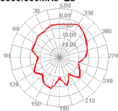
5400.000MHz H
