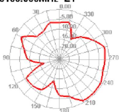
5100.000MHz E1
