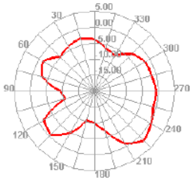
5600.000MHz E1
