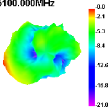
5100.000MHz E1
