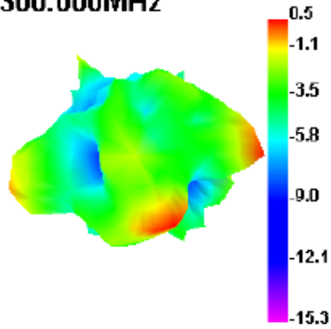
5300.000MHz E1
