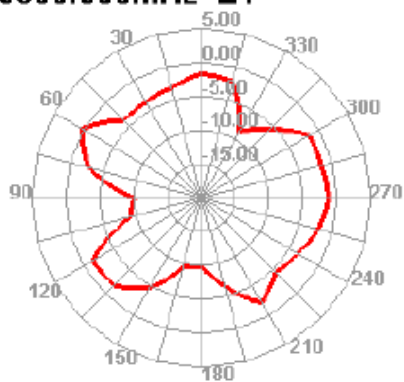
5300.000MHz E1
