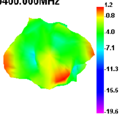
5400.000MHz E1
