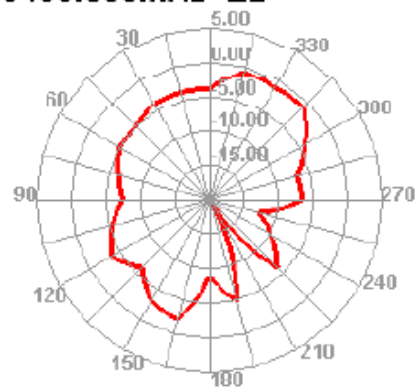
5400.000MHz E2
