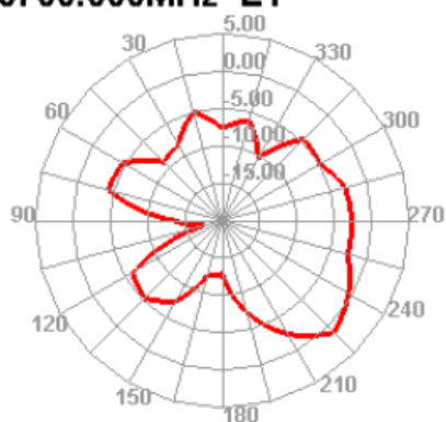
5700.000MHz E1
