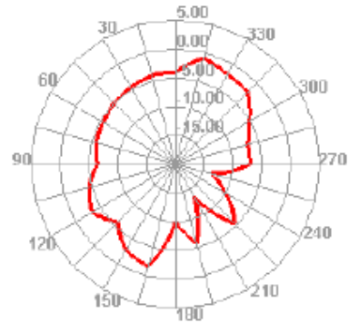
5600.000MHz E2
