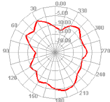
5200.000MHz H
