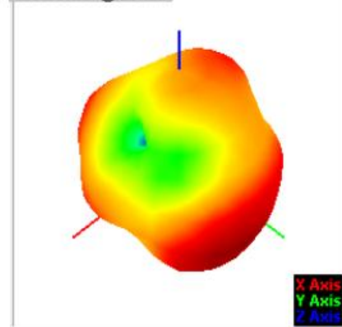
2430.00MHz@T45P45
