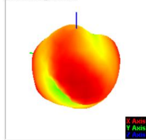
2440.00MHz@T45P200
