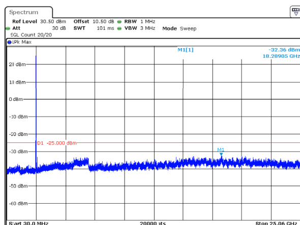
20MHz_Low_QPSK_1@0 -32.36dBm
