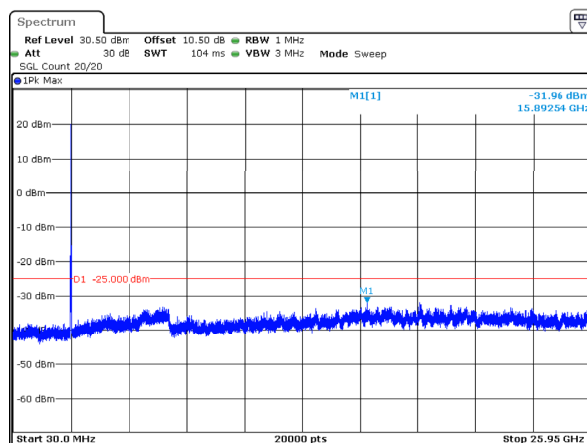
10MHz_Middle_QPSK_50@0 -31.96dBm
