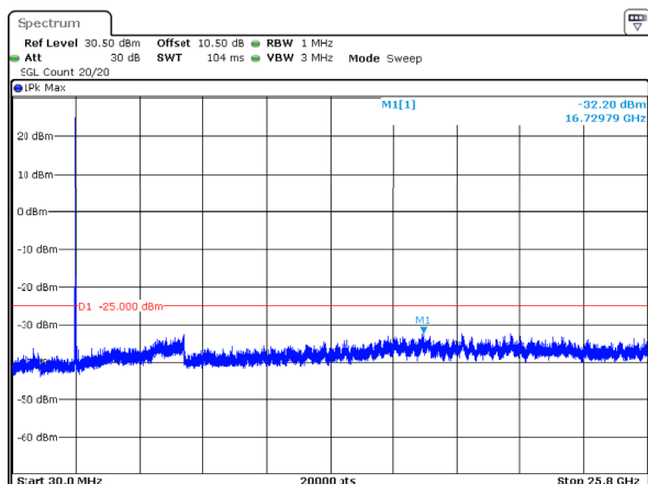
20MHz_Low_QPSK_1@0 -32.20dBm
