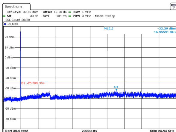
10MHz_Middle_QPSK_1@0 -32.39dBm
