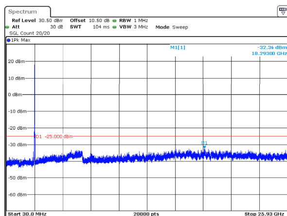
20MHz_Middle_QPSK_100@0 -32.36dBm
