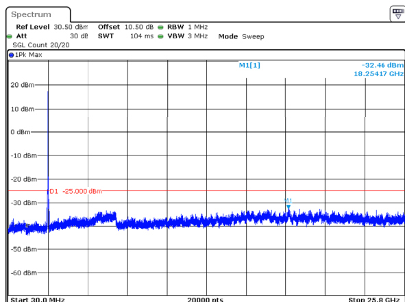
20MHz_Low_QPSK_100@0 -32.46dBm
