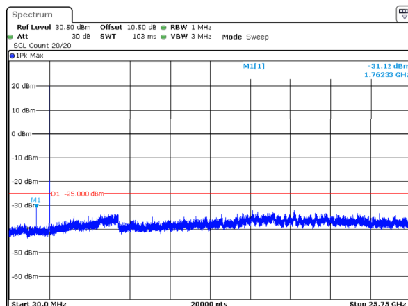
10MHz_Low_QPSK_50@0 -31.12dBm
