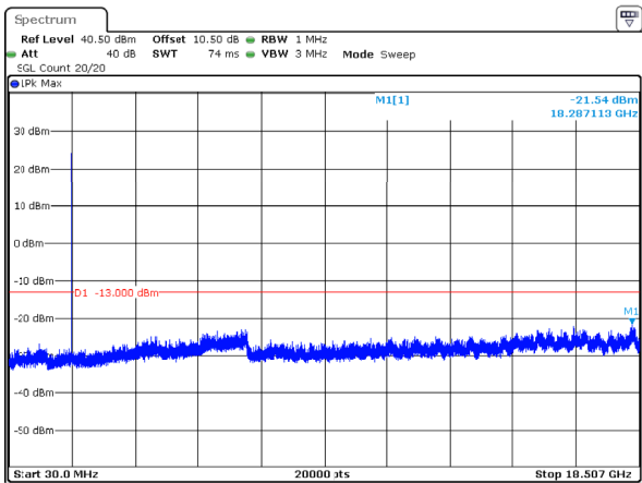
1.4MHz_Low_QPSK_1@0
