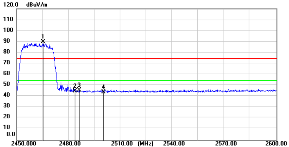
11ax(HE20)_TX_CH_11_Horizontal_Peak
