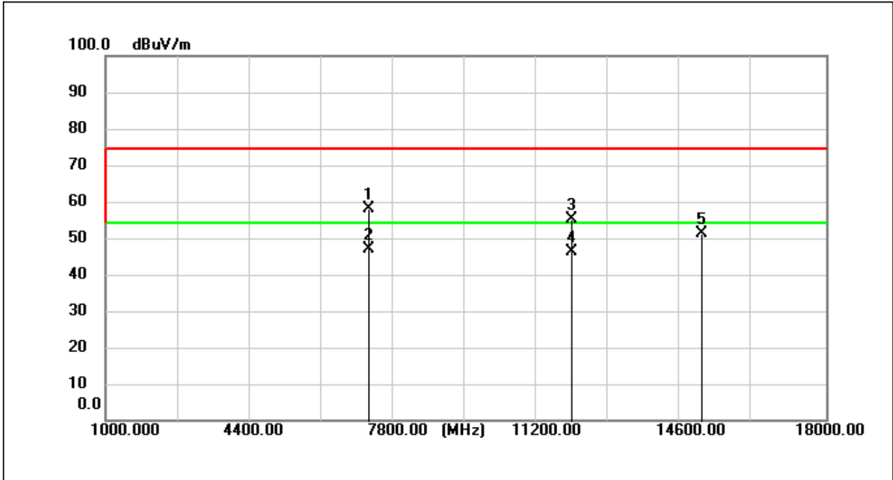
BLE_2M_TX_CH_39_Verical
