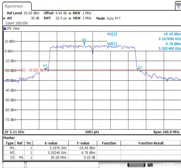
11AC80SISO-Ant1-5210
