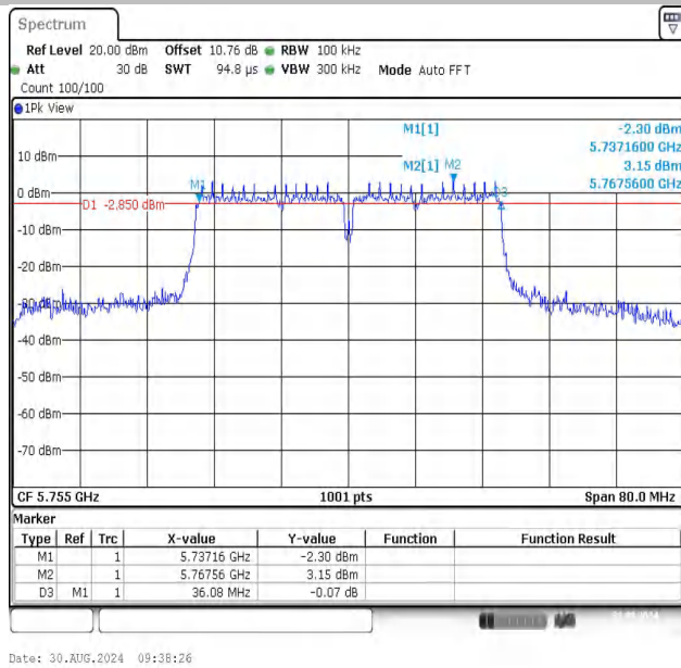
11N40SISO-Ant1-5755-PASS
