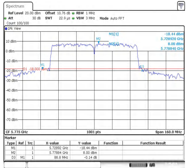
11AC80SISO-Ant1-5775
