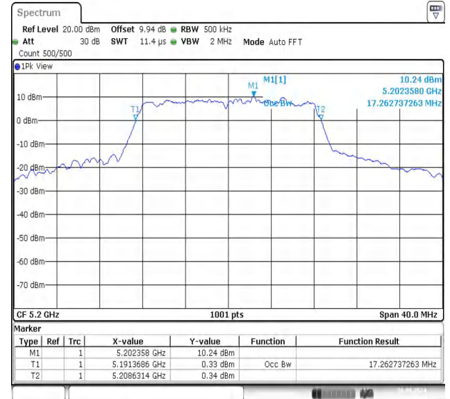
11A-Ant1-5200
