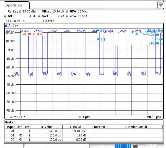
NTNV-11A-Ant1-5745
