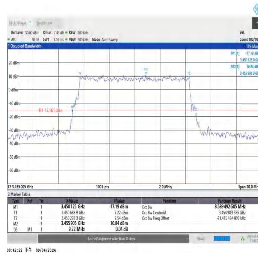
NTNV_N77-3450-3550_PC3_30_10_L_TID3_Ant
