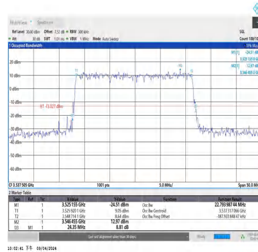
NTNV_N77-3450-3550_PC3_30_25_H_TID1_Ant
