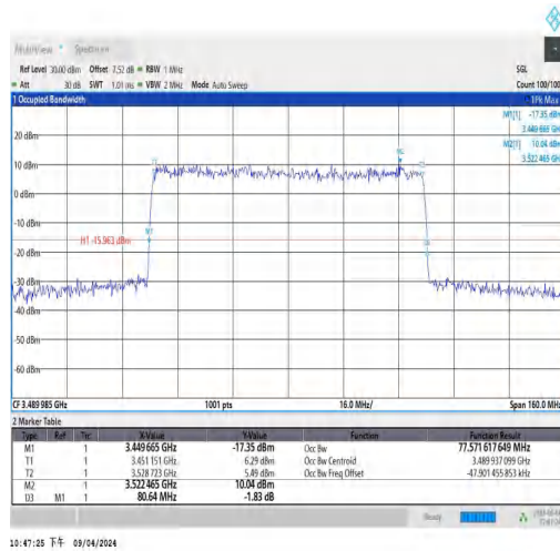
NTNV_N77-3450-3550_PC3_30_80_L_TID6_Ant
