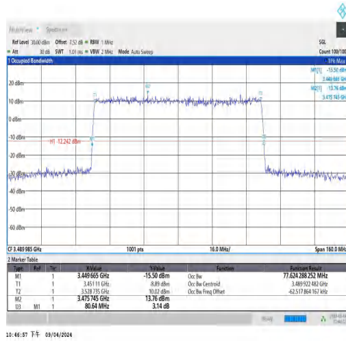
NTNV_N77-3450-3550_PC3_30_80_L_TID4_Ant
