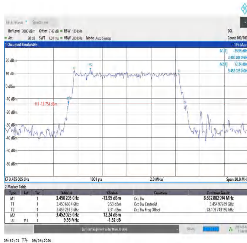
NTNV_N77-3450-3550_PC3_30_10_L_TID2_Ant
