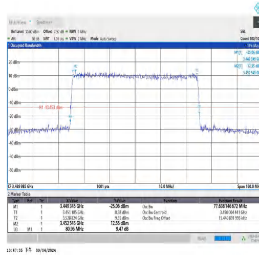
NTNV_N77-3450-3550_PC3_30_80_L_TID5_Ant
