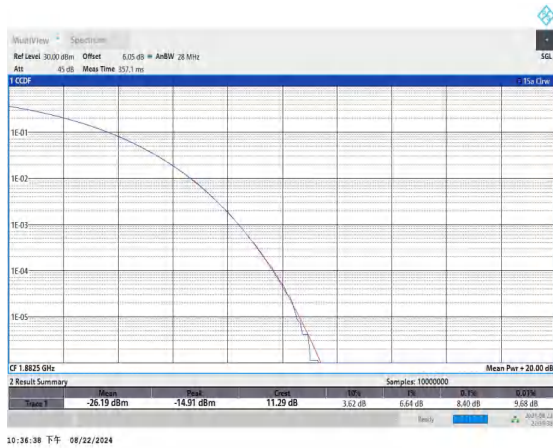
Band25-20MHz-QPSK-26365-1RB#0-PASS
