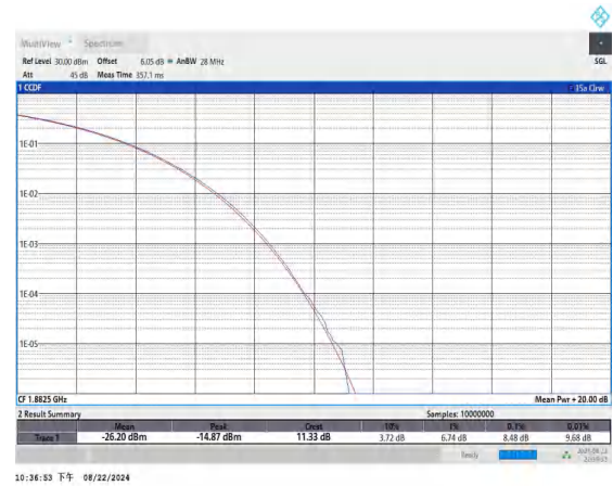
Band25-20MHz-16QAM-26365-100RB#0-PASS
