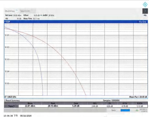
Band25-5MHz-QPSK-26365-25RB#0-PASS
