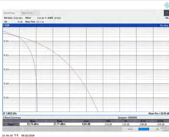
Band25-5MHz-QPSK-26365-1RB#0-PASS
