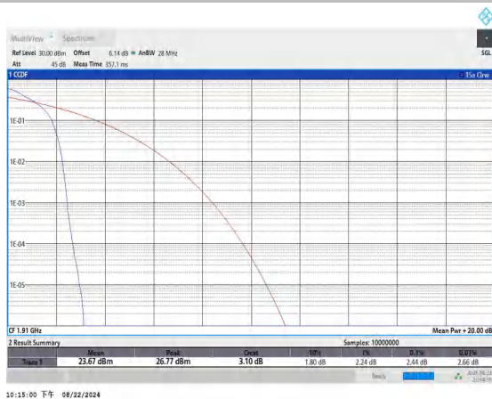
Band25-10MHz-QPSK-26640-1RB#0-PASS
