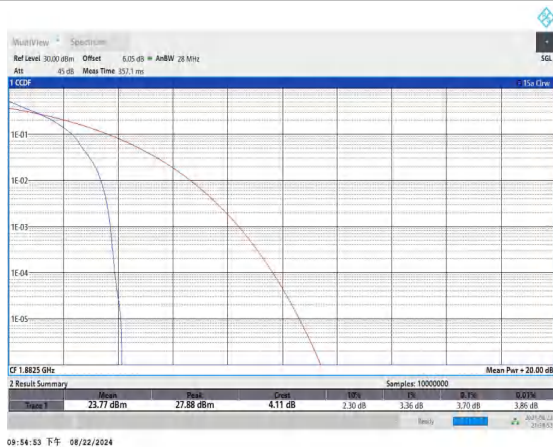
Band25-3MHz-QPSK-26365-1RB#0-PASS
