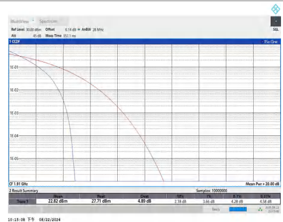
Band25-10MHz-QPSK-26640-50RB#0-PASS
