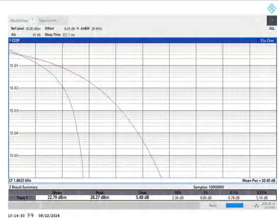
Band25-10MHz-QPSK-26365-50RB#0-PASS
