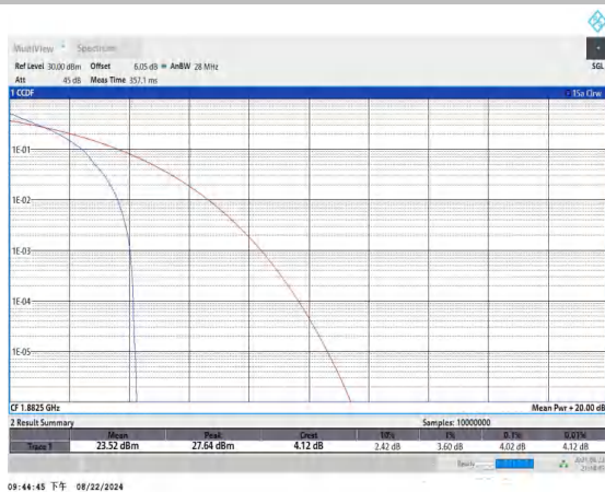
Band25-1.4MHz-QPSK-26365-1RB#0-PASS
