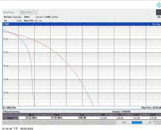
Band25-10MHz-QPSK-26365-1RB#0-PASS
