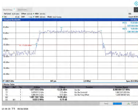
Band25-10MHz-16QAM-26365-50RB#0-PASS
