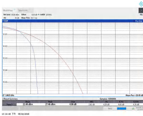
Band25-10MHz-16QAM-26365-1RB#0-PASS
