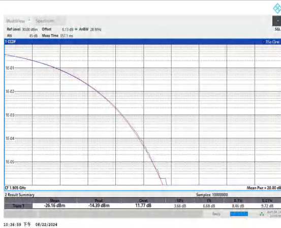
Band25-20MHz-QPSK-26590-1RB#0-PASS
