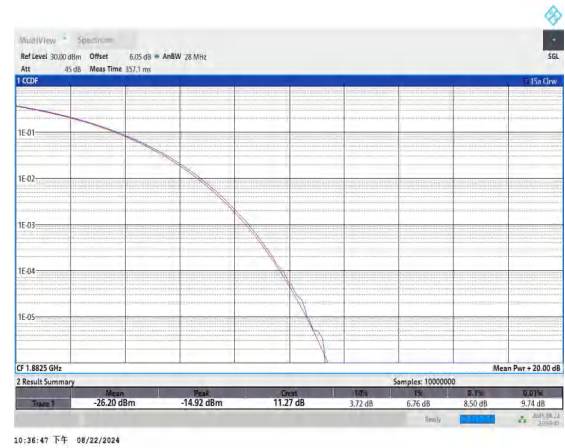
Band25-20MHz-QPSK-26365-100RB#0-PASS
