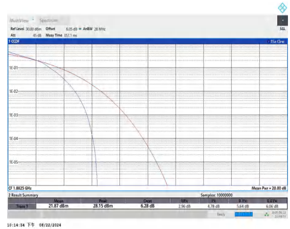
Band25-10MHz-16QAM-26365-50RB#0-PASS
