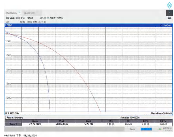
Band25-3MHz-QPSK-26365-15RB#0-PASS
