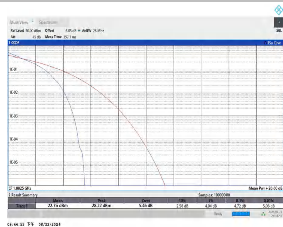
Band25-1.4MHz-QPSK-26365-6RB#0-PASS
