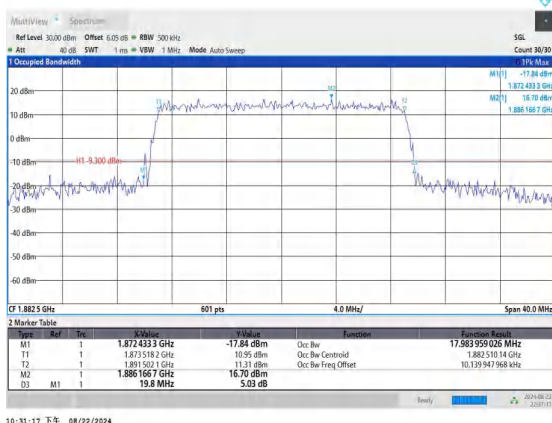
Band25-20MHz-16QAM-26365-100RB#0-PASS
