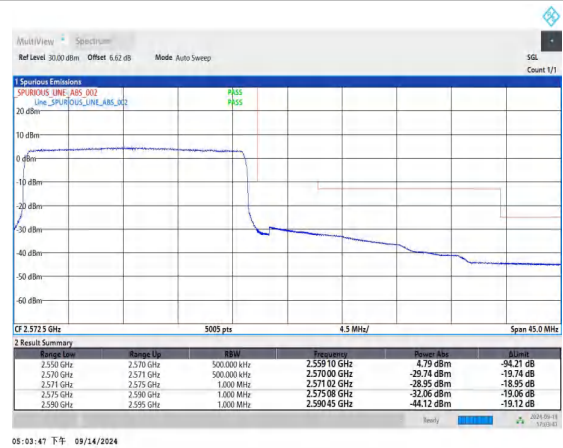
Band7_20MHz_QPSK_21350_100RB#0
