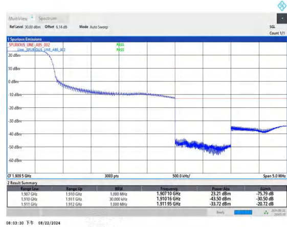
Band2_3MHz_QPSK_19185_1RB#0
