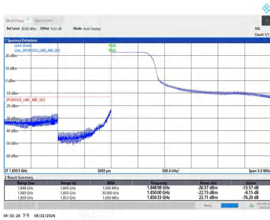
Band2_3MHz_QPSK_18615_1RB#0
