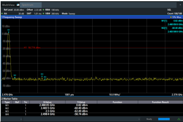
BLE 1M: Band Edge, Right Side
