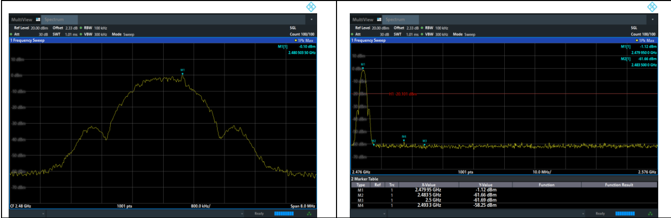
BLE 2M: Band Edge, Right Side
