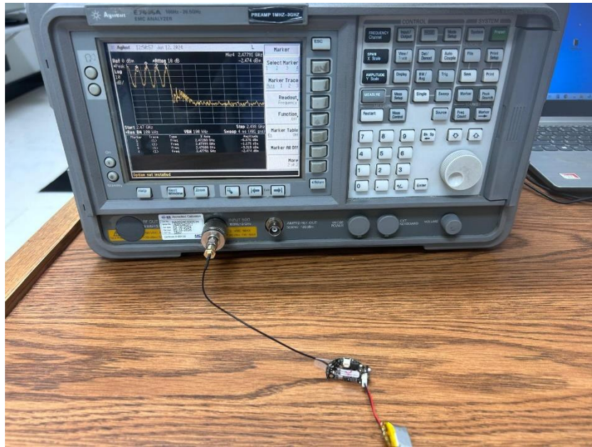
CE Test Setup
