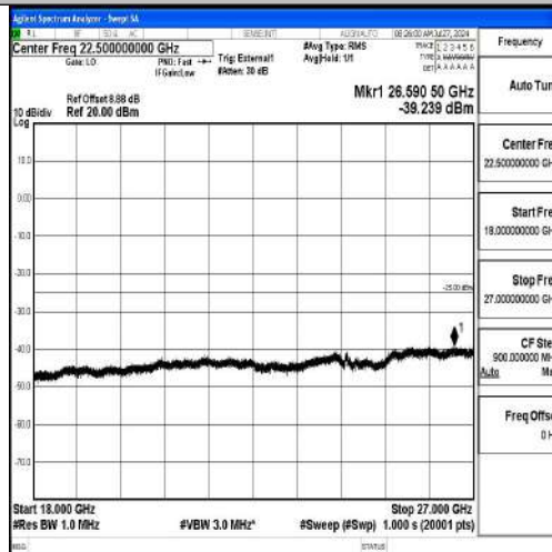
Band41-20MHz-16QAM-41490-1RB#0-18000~27000-PASS
