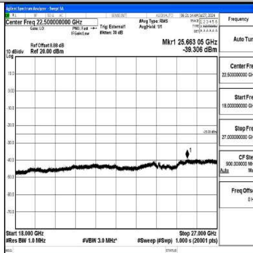
Band41-5MHz-16QAM-41565-1RB#0-18000~27000-PASS
