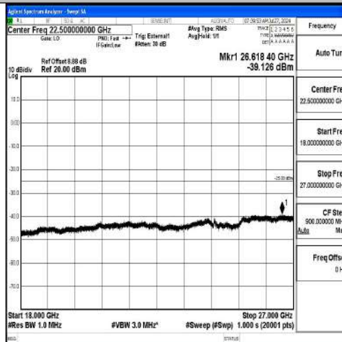
Band41-15MHz-16QAM-41515-1RB#0-18000~27000-PASS
