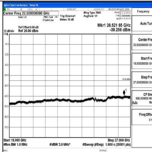
Band41-20MHz-QPSK-41490-1RB#0-18000~27000-PASS
