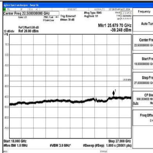
Band41-15MHz-16QAM-39725-1RB#0-18000~27000-PASS
