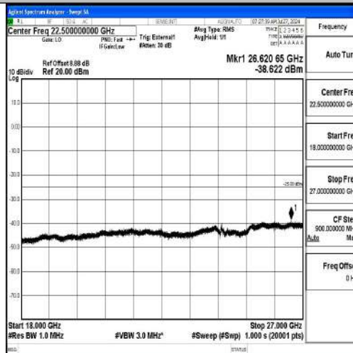
Band41-15MHz-QPSK-39725-1RB#0-18000~27000-PASS
