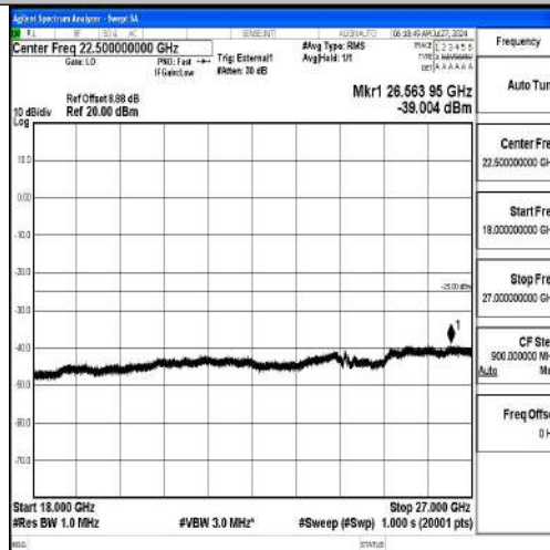
Band41-5MHz-QPSK-41565-1RB#0-18000~27000-PASS
