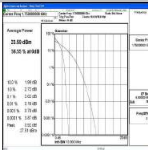
Band4-10MHz-QPSK-20350-1RB#0-PASS
