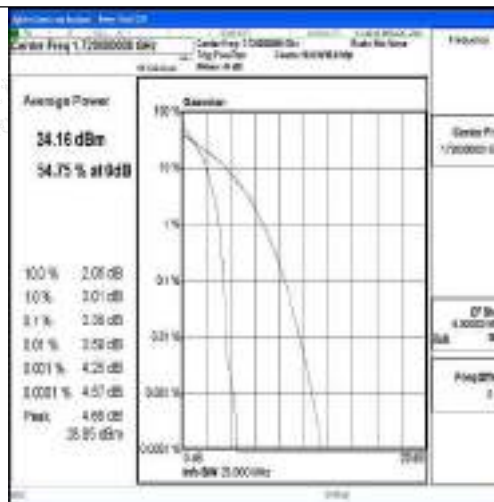
Band4-20MHz-QPSK-20050-1RB#0-PASS
