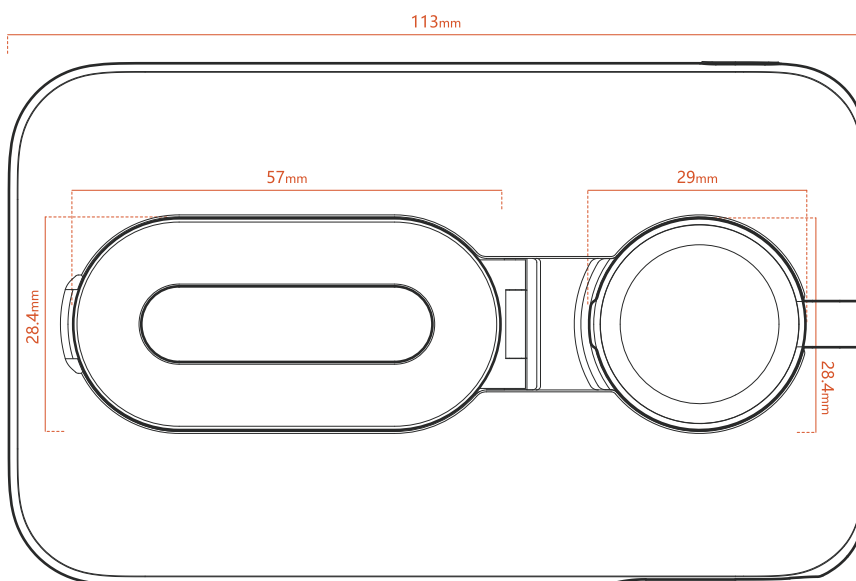
后视图 BACK
