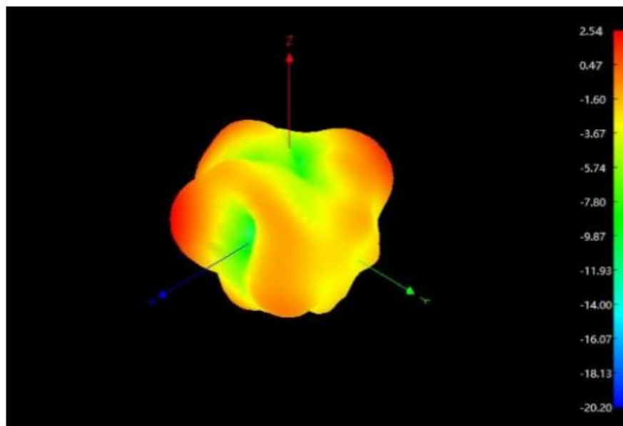
2480MHz 3D
