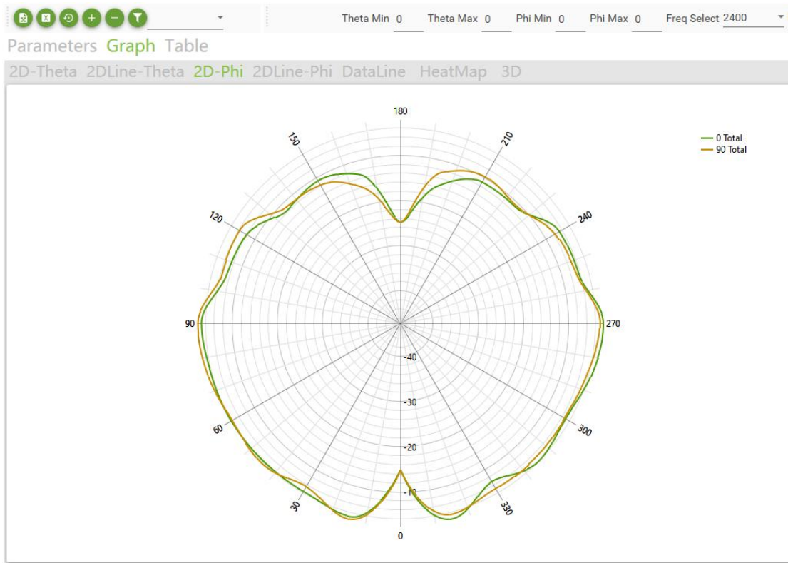
Phi=0°&Phi=90°_2400MHz
