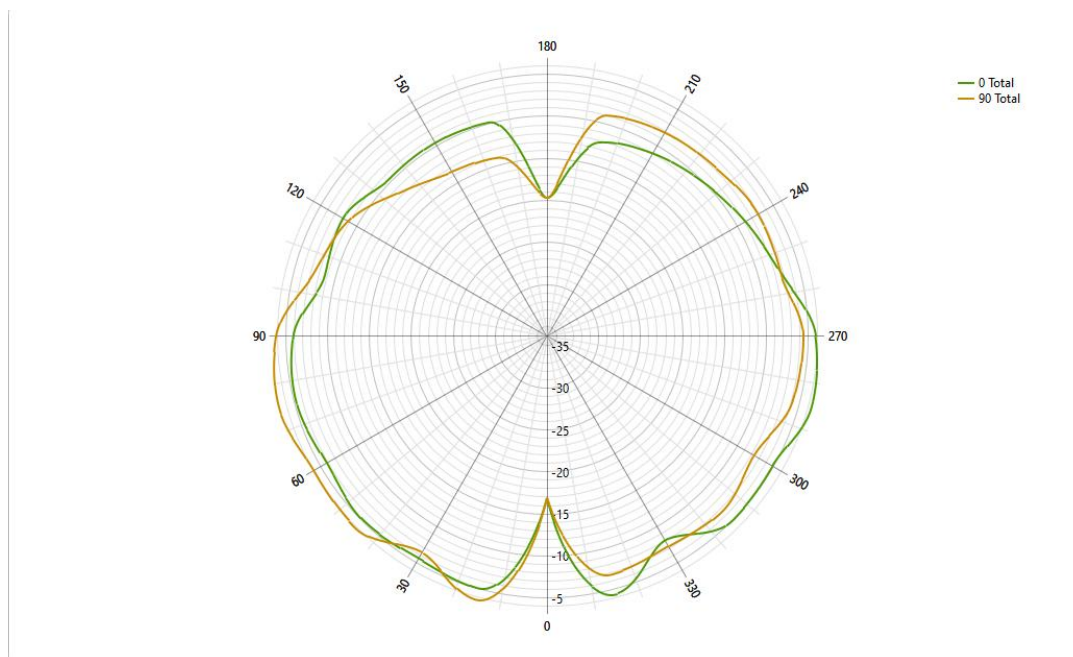
Phi=0°&Phi=90°_2500MHz
