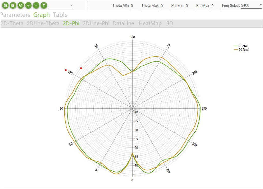
Phi=0°&Phi=90°_2460MHz
