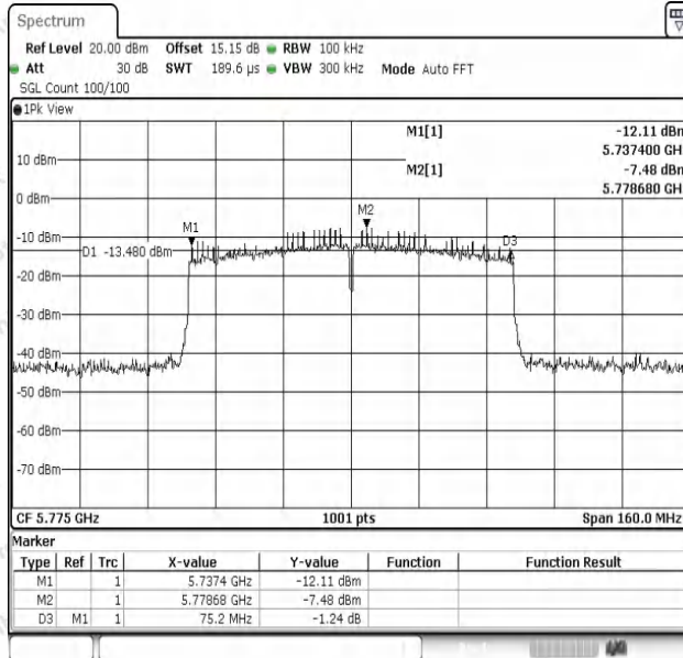
11AC80SISO-Ant1-5775-PASS
