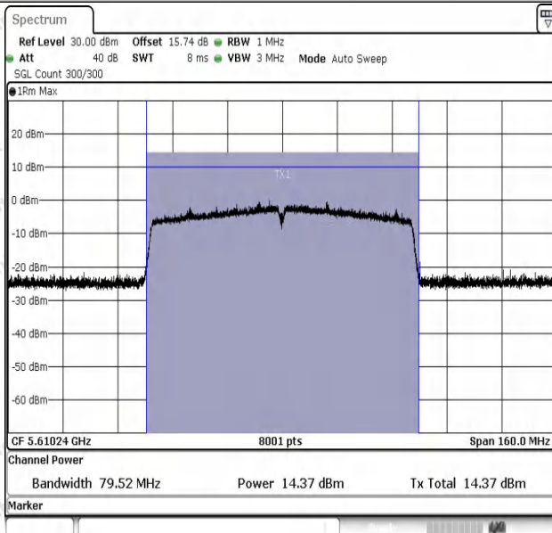
11AC80SISO-Ant1-5610-PASS
