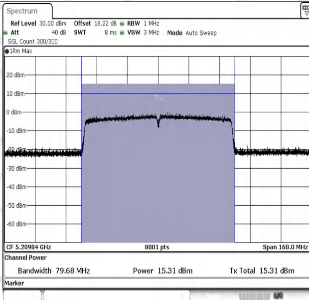
11AC80SISO-Ant1-5210-PASS
