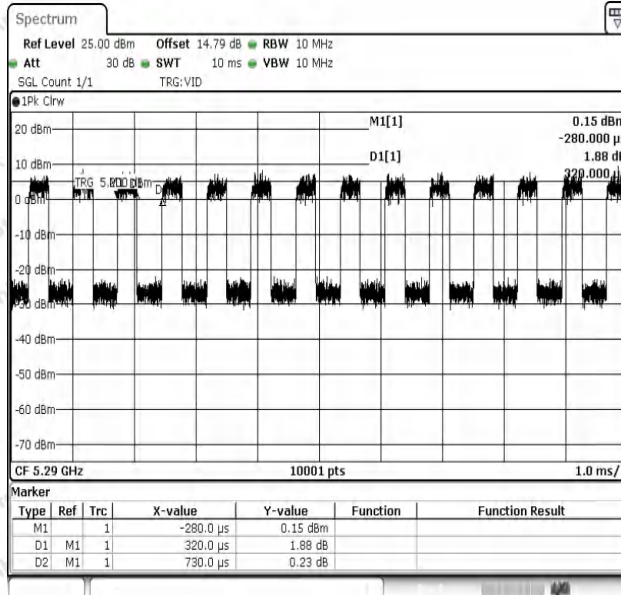
NTNV-11AC80SISO-Ant1-5290
