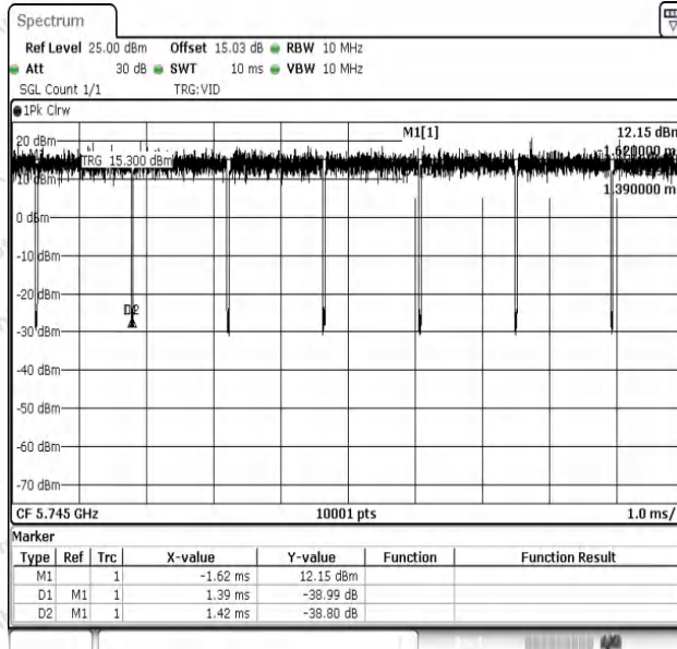
NTNV-11A-Ant1-5745
