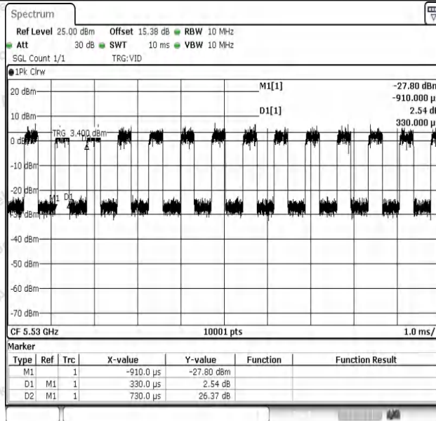
NTNV-11AC80SISO-Ant1-5530
