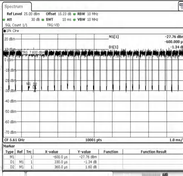
NTNV-11AC80SISO-Ant1-5610
