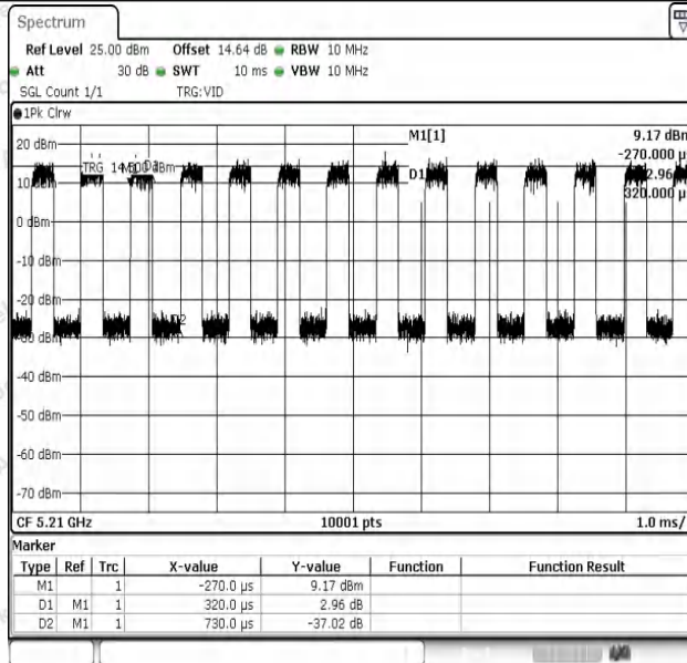
NTNV-11AC80SISO-Ant1-5210
