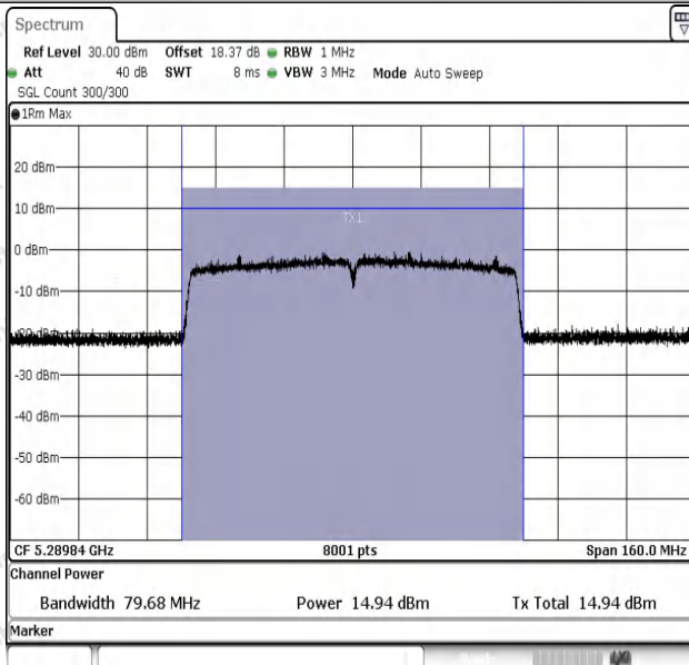
11AC80SISO-Ant1-5290-PASS
