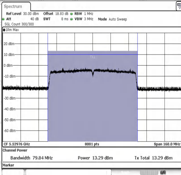
11AC80SISO-Ant1-5530-PASS
