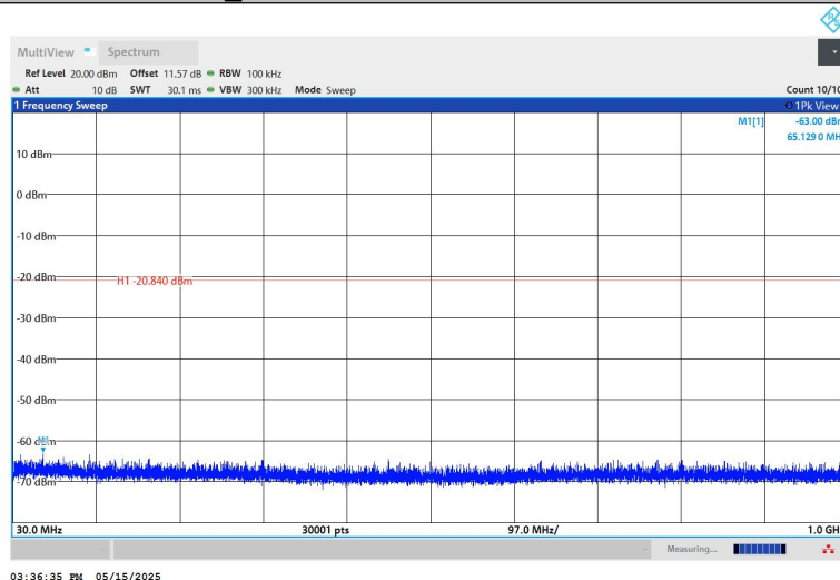
BLE_2M-Ant1-2440-30~1000-PASS
