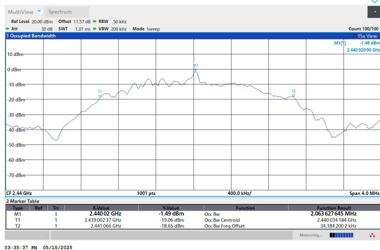
BLE_2M-Ant1-2440
