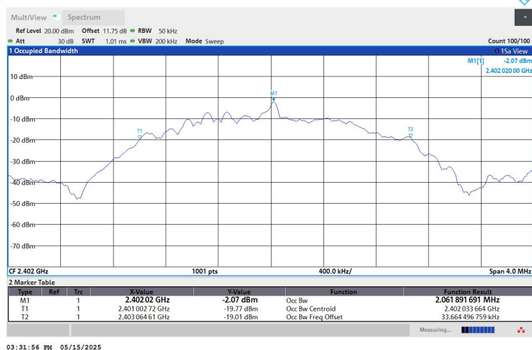
BLE_2M-Ant1-2402
