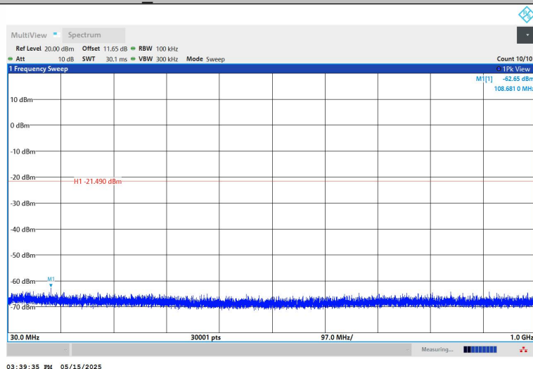
BLE_2M-Ant1-2480-30~1000-PASS
