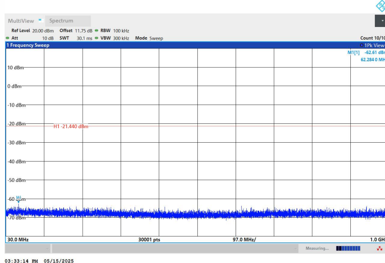
BLE_2M-Ant1-2402-30~1000-PASS
