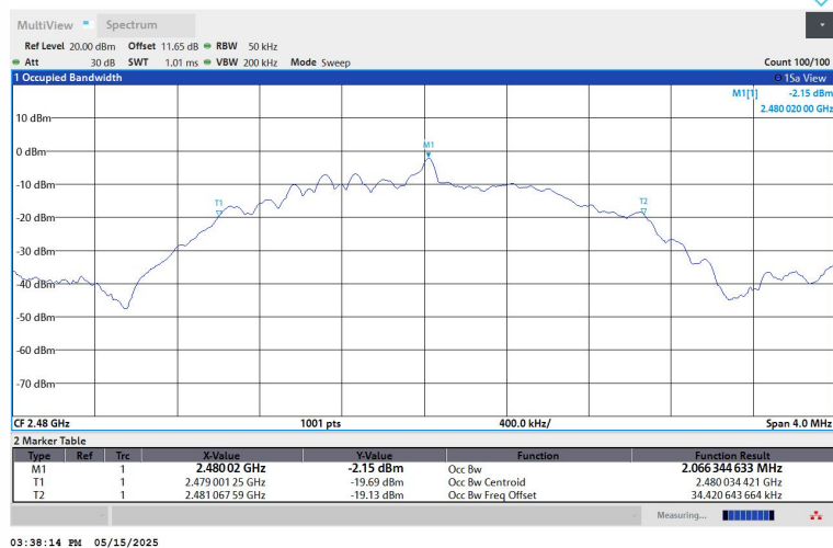
BLE_2M-Ant1-2480
