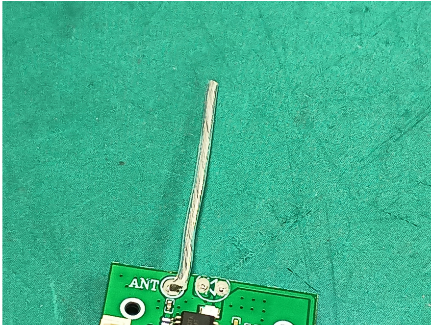
RX ANT
