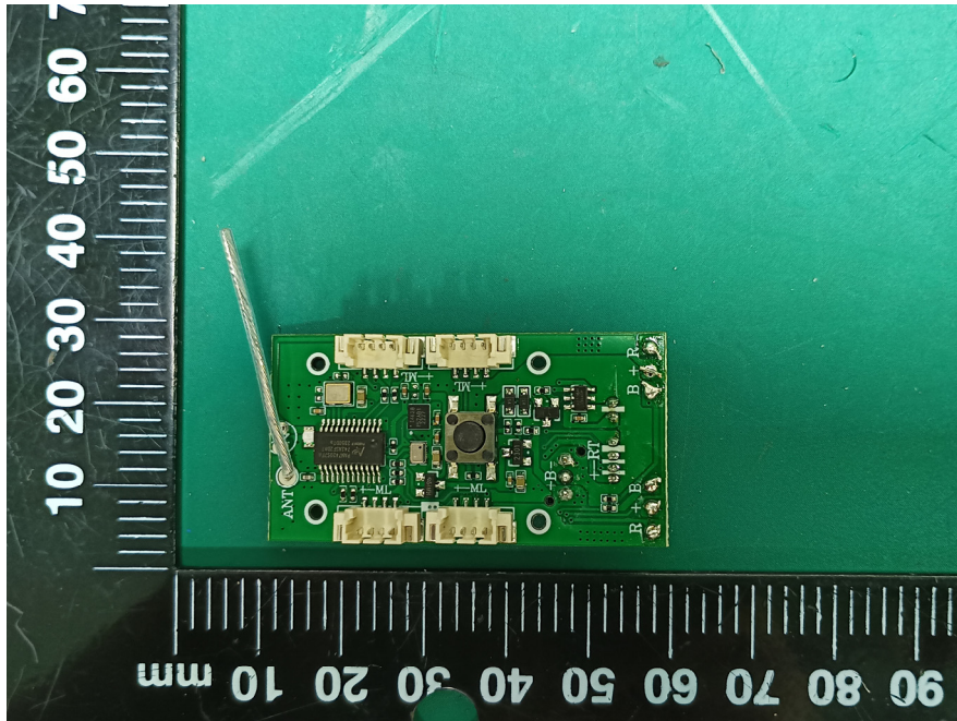
RX Module
