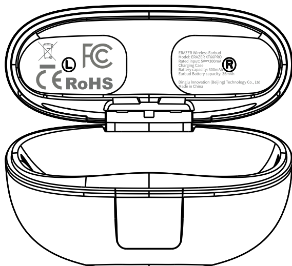
上盖内腔
