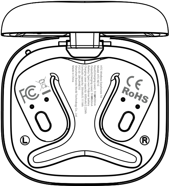
底盒内腔 镭雕
