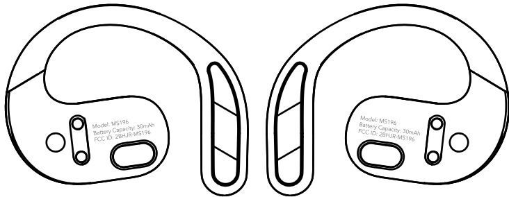
耳机内侧 丝印
