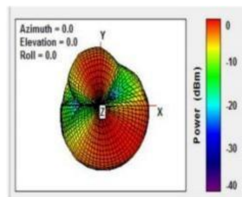
RadiatXion Pattern
