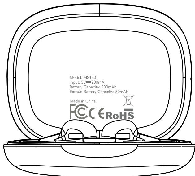
上盖内腔
